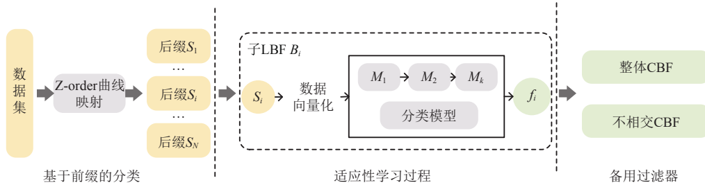
图 11 PA-LBF 索引结构 [34]
