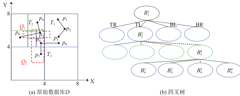
图 6 RL4QDTS 的运行示例 [15]
