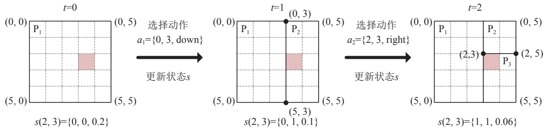
图 5 DRL-Partitioner 的运行示例 [21]
