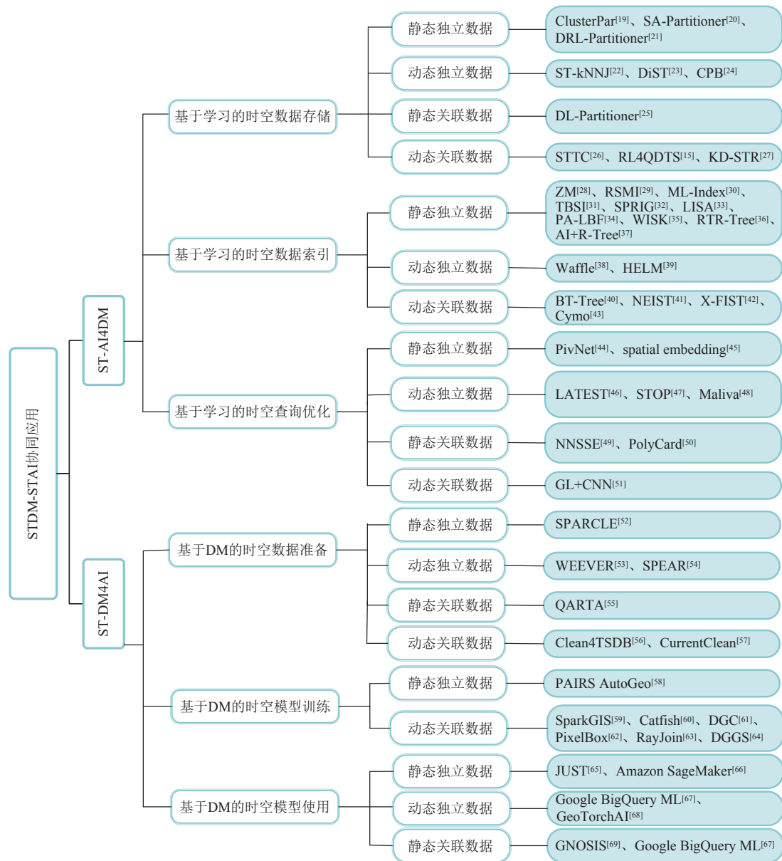
图2 ST-AI4DM 和 ST-DM4AI 的研究分类
