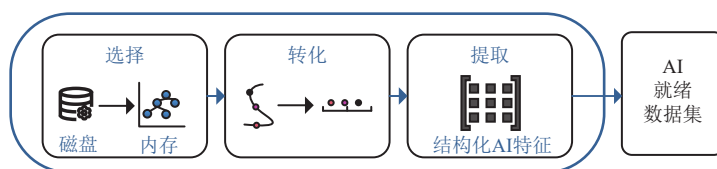
图 20 ST4ML 三阶段示意图
