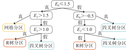
图 4 决策树模型示意图
