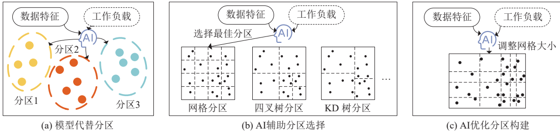
图3 基于学习的时空分区方法
