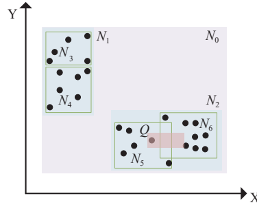
图 12 具有重叠节点的 R 树示例
