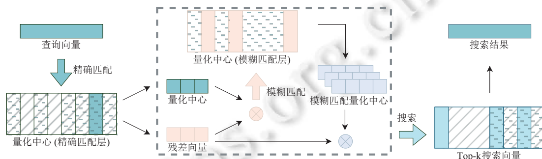
图 3 基于权重向量量化的索引结构
