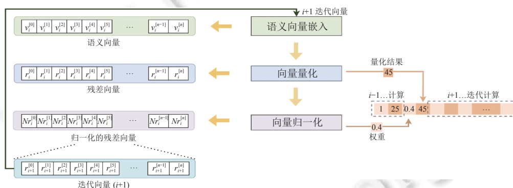
图 2 权重优化的向量量化表征
