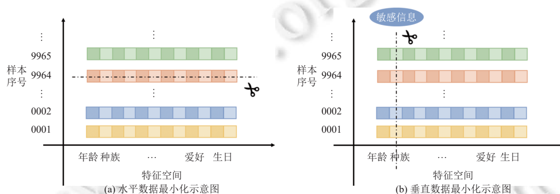
图2 数据最小化分类系统与工作机理
