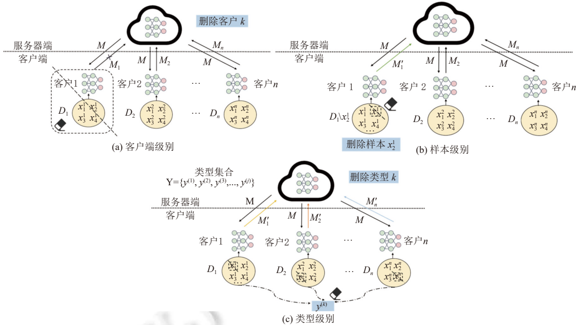
图5 联邦忘却学习框架示意图
