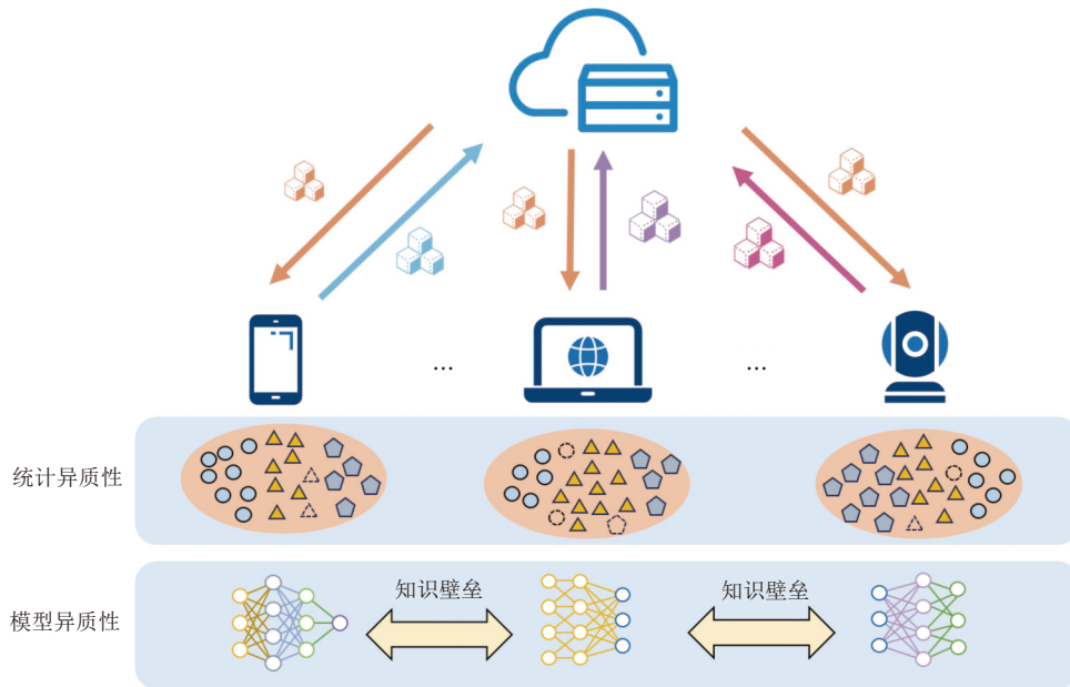
图4 个性化联邦学习框架示意图
