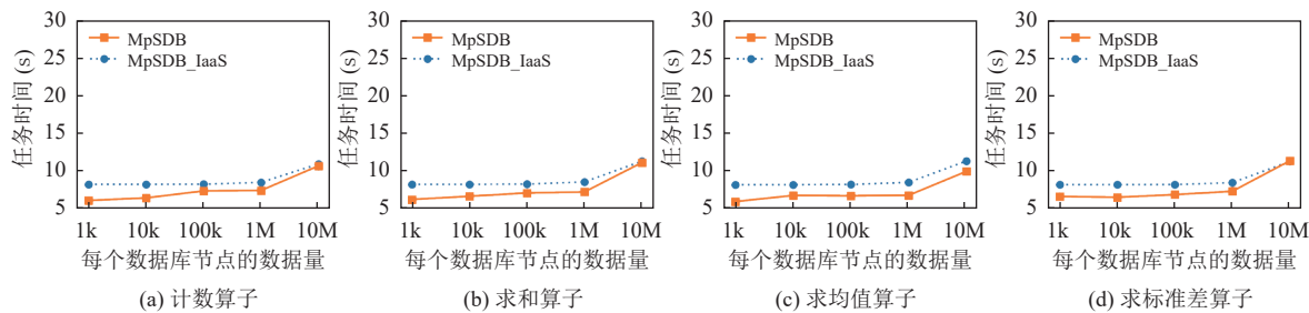
图 12 纵向数据结构下查询计算任务性能比较 (TPC-H 数据集)
