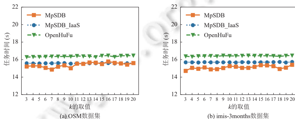
图10 横向数据结构下 k 的取值对 kNN 查询算子性能的影响
