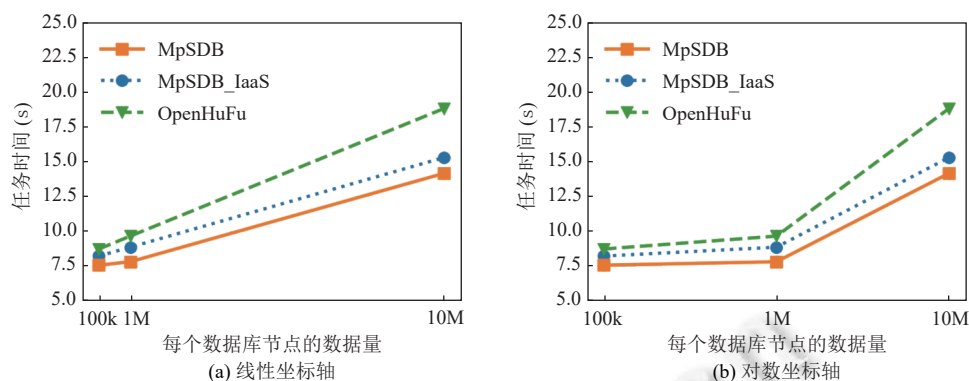
图9 x 轴形式对算子查询时间变化的影响
