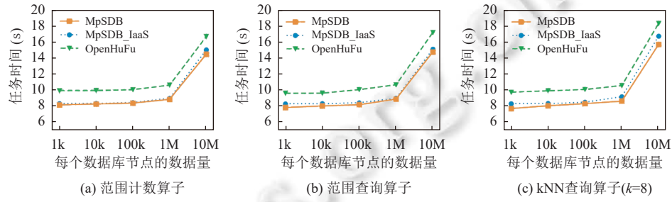
图6 横向数据结构下查询任务性能比较 (OSM 数据集)
