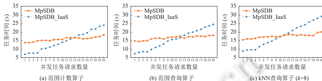
图 19 用户任务数量的系统扩展性实验 (imis-3months 数据集)
