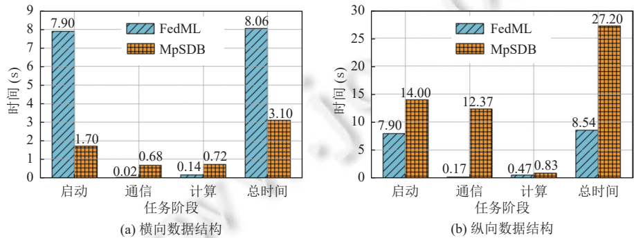
图 13 Linear 模型训练的时间分解
