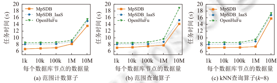
图8 横向数据结构下查询任务性能比较 (imis-3months 数据集)
