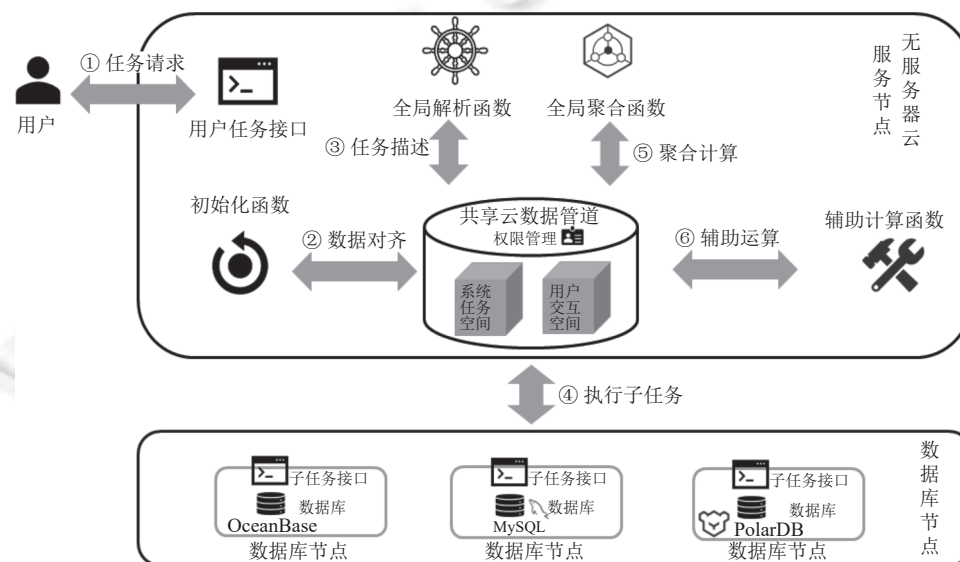
图 2 多方数据库安全查询任务运行流程
