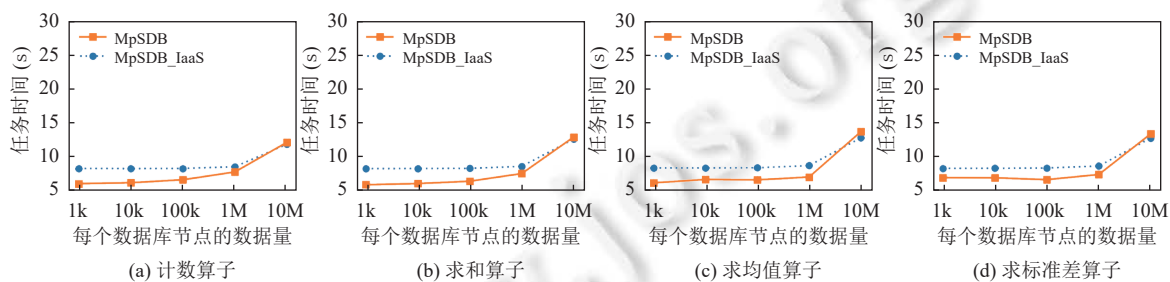
图11 纵向数据结构下查询计算任务性能比较(NYU taxi 数据集)
