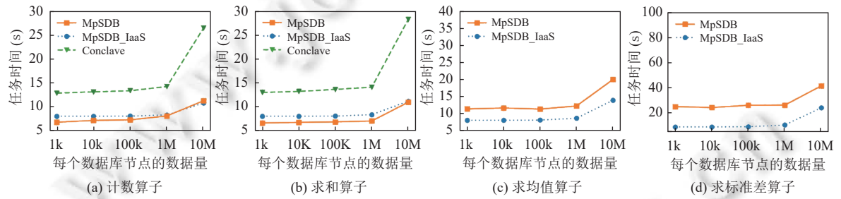
图7 横向数据结构下查询任务性能比较 (TPC-H 数据集)
