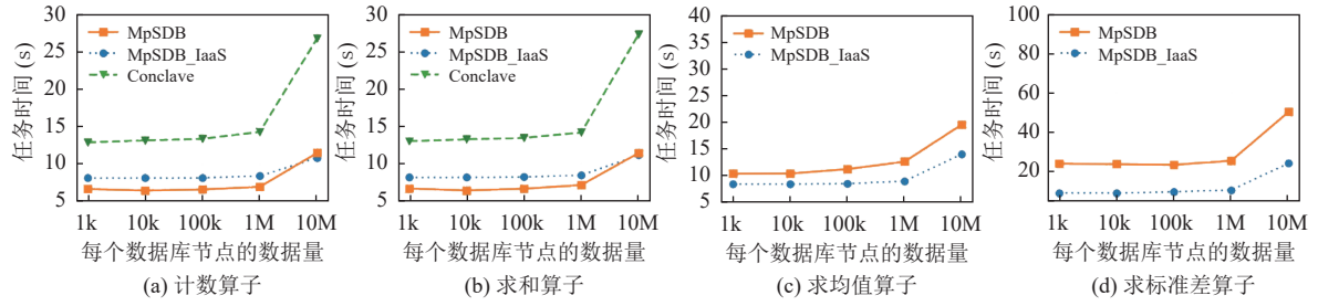
图5 横向数据结构下查询任务性能比较 (NYU taxi 数据集)
