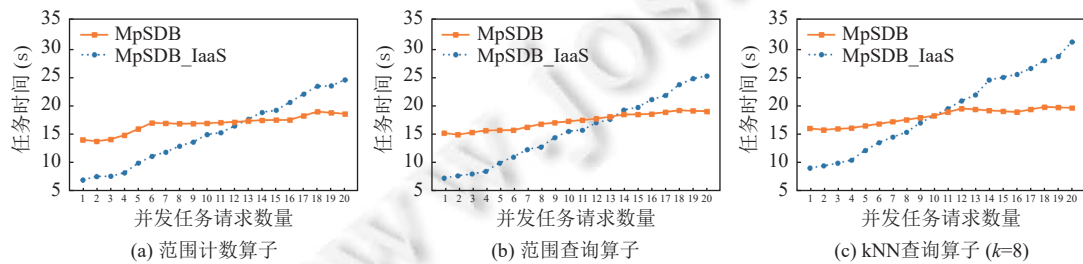
图 18 用户任务数量的系统扩展性实验 (OSM 数据集)
