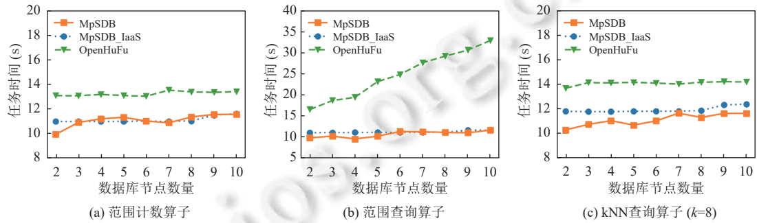
图 17 数据库节点数量的系统扩展性实验 (imis-3months 数据集)
