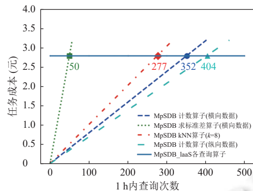
图 4 查询任务成本随查询频次变化图
