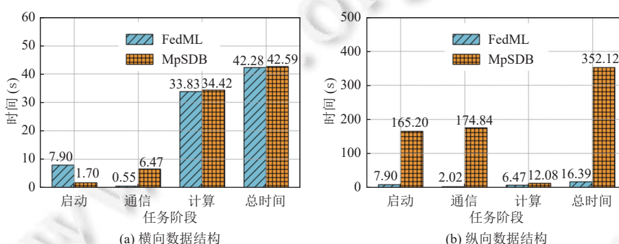
图 15 CNN 模型训练的时间分解
