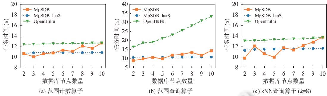
图 16 数据库节点数量的系统扩展性实验 (OSM 数据集)
