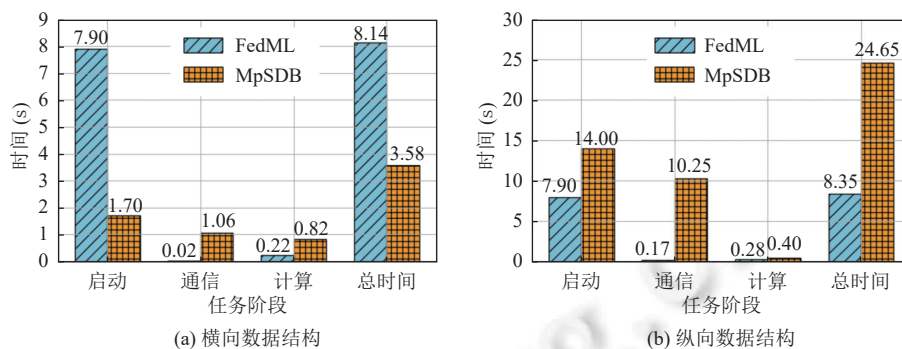
图 14 MLP 模型训练的时间分解
