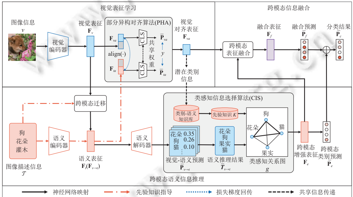
图 2 基于跨模态信息推理和融合的图片分类框架 CMIF
