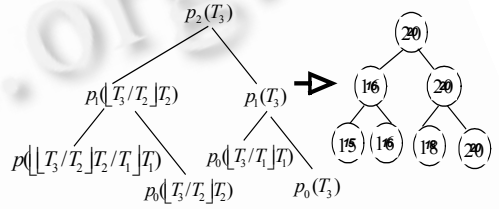
Fig.3 Bintree expression of p_2(T_3) in Example 1 图 3 例 1 中 p_2(T_3) 的二叉树表示
