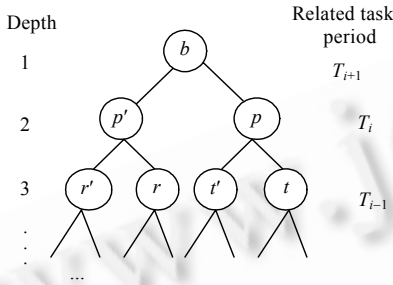
Fig.2 Bintree expression of RM schedulability space p_i(b) 图 2 任务 RM 调度空间 p_i(b) 的二叉树
