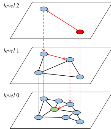
图 2 HNSW 索引查询过程
