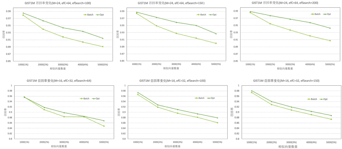
图 10 GIST1M 数据集的平均召回率
