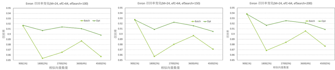
图 12 Enron 数据集的平均召回率
