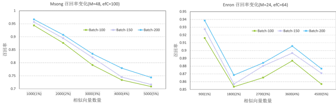
图 5 Msong( M=48 , efC=100 ) 和 Enron( M=24 , efC=64 ) 数据集上的平均召回率
