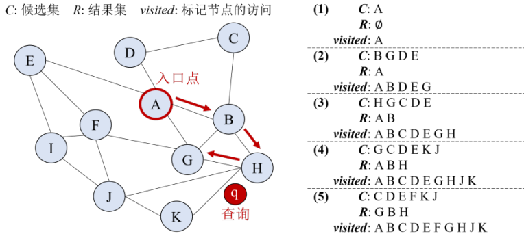
图 1 图向量索引的查询过程
