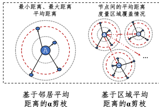
图 7 局部过度致密区域的识别方法
