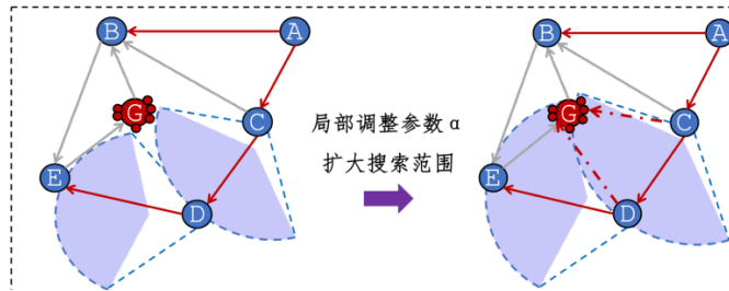
图 8 修正的启发式剪枝规则
