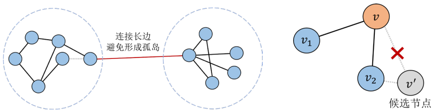
图 3 索引的孤岛效应(左)以及启发式剪枝规则(右)
