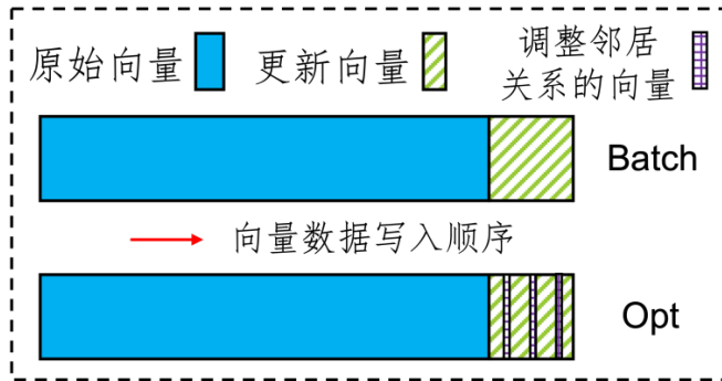
图9 数据写入场景的实验负载
