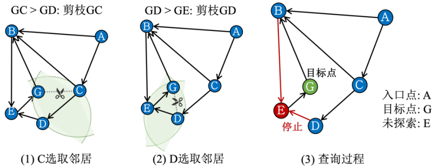
图 6 启发式规则造成的过度剪枝
