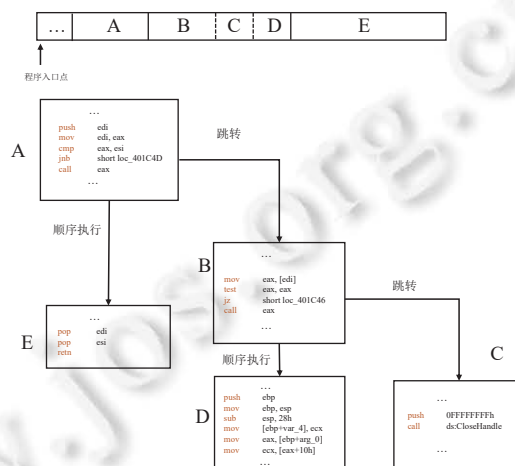
图 2 执行导向的操作码序列提取
