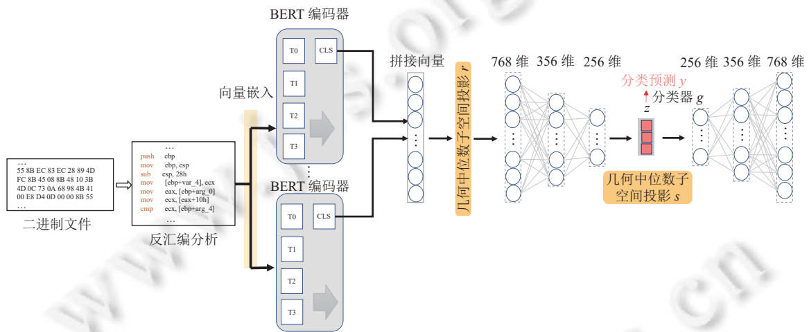
图 1 基于 BERT 和瓶颈自编码器的恶意软件分类模型系统架构
