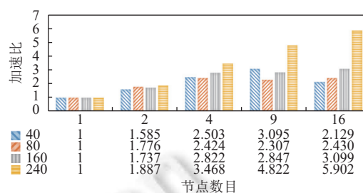
图 8 交通仿真执行加速比分析图
