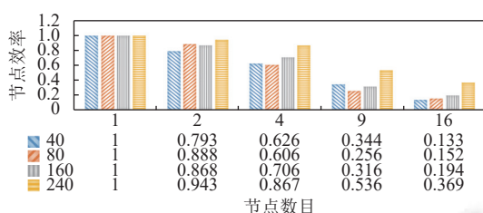
图 9 交通仿真执行并行效率分析图
