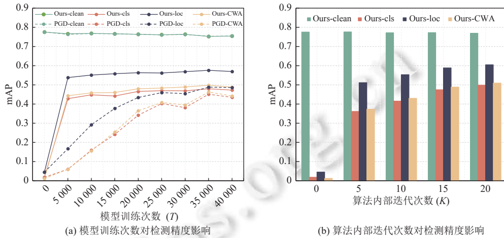
图 3 模型训练次数 ( T ) 和算法内部迭代次数 ( K ) 对 PGD 和本文方法所训练模型的检测精度影响
