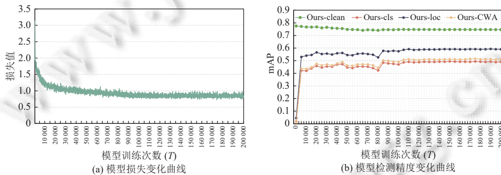
图 4 长期训练下模型的训练损失和检测精度变化趋势图
