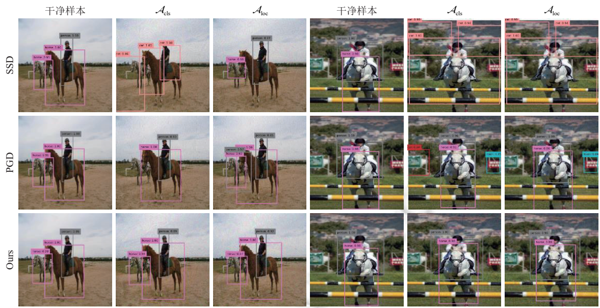
图2 SSD、PGD 和本文方法所训练模型的检测结果
