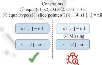
图 7 L2-3 代码检查工具规则
