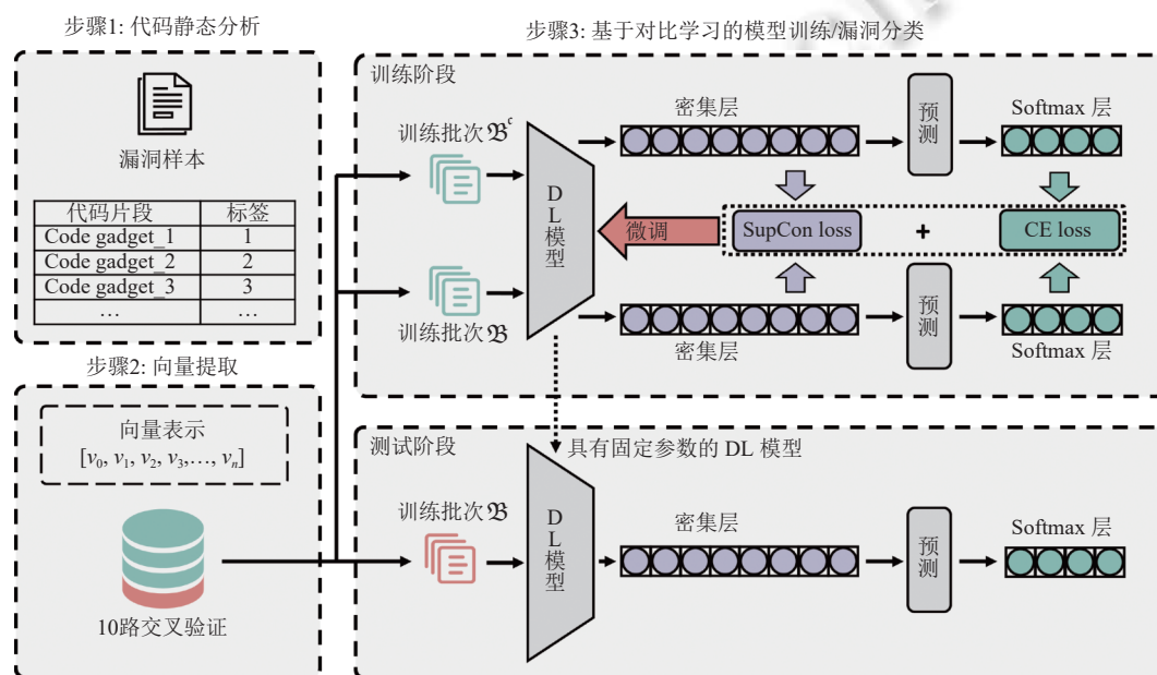
图 5 VulFewShot 的系统概述
