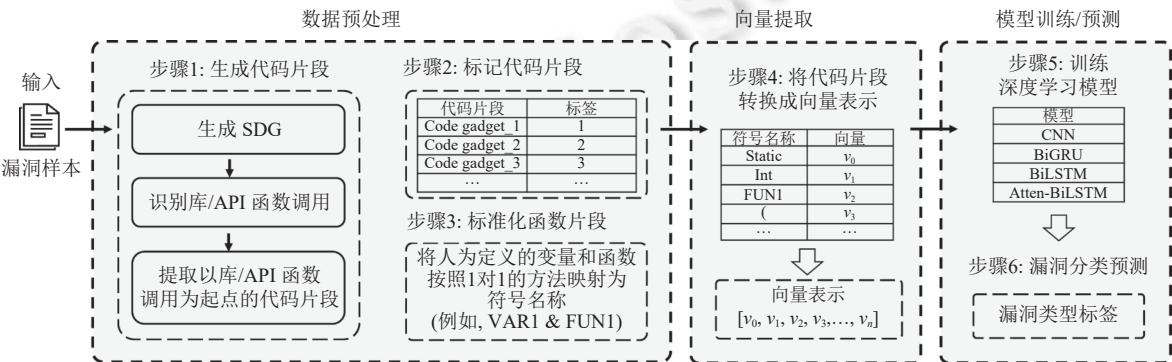
图 1 漏洞分类的一般过程
