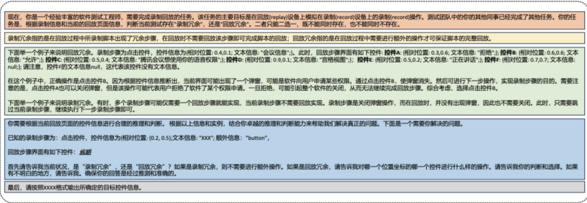
图 5 提示词样例
