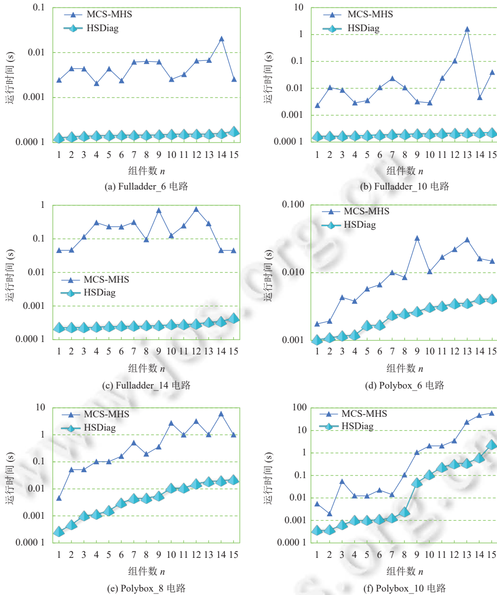
图8 HSDiag 与 MCS-MHS 算法在 Polybox, Fulladder 电路实验比较
