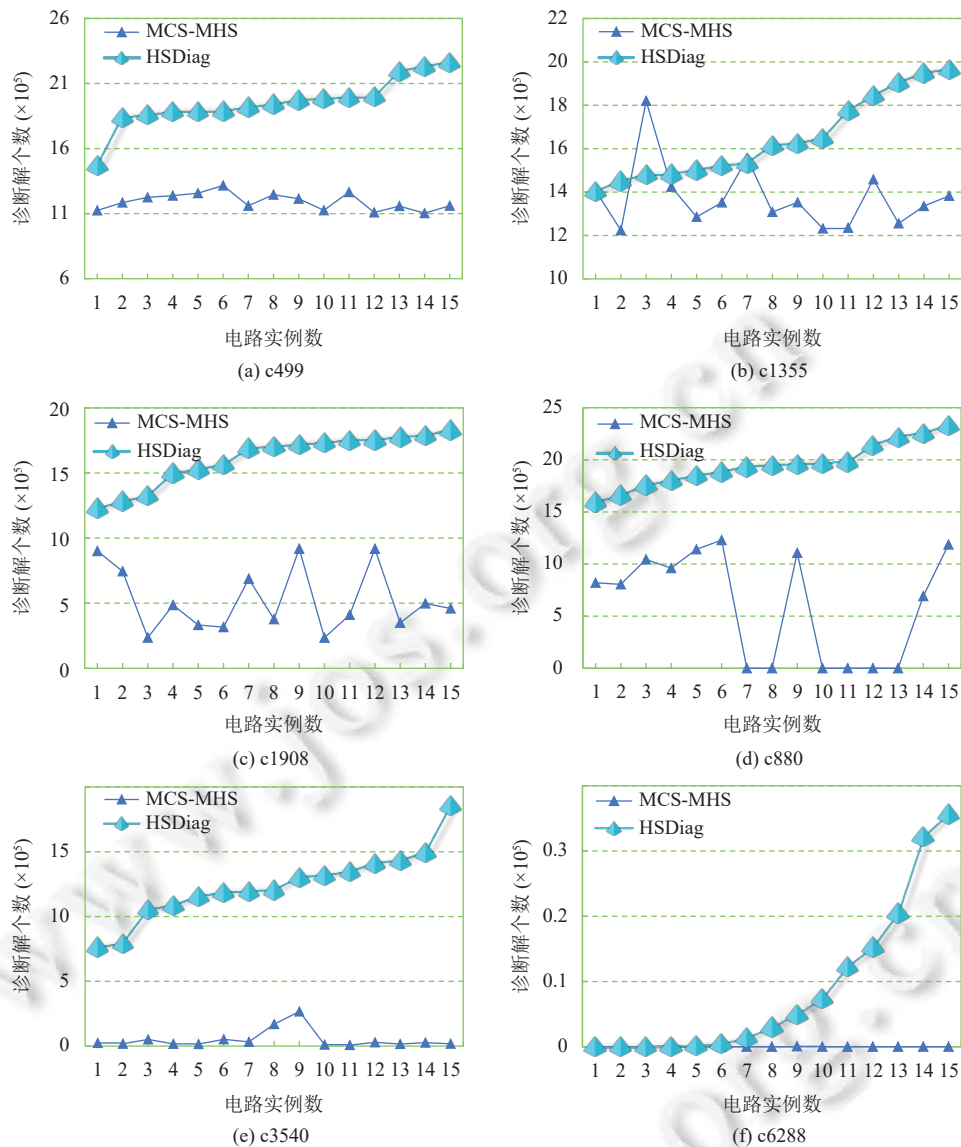
图9 HSDiag 与 MCS-MHS 算法在 ISCAS-85 电路实验比较
