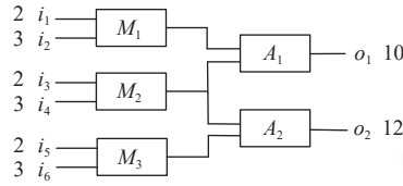
图 2 乘法加法器电路实例
