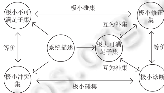
图 4 系统描述到候选诊断关系图
