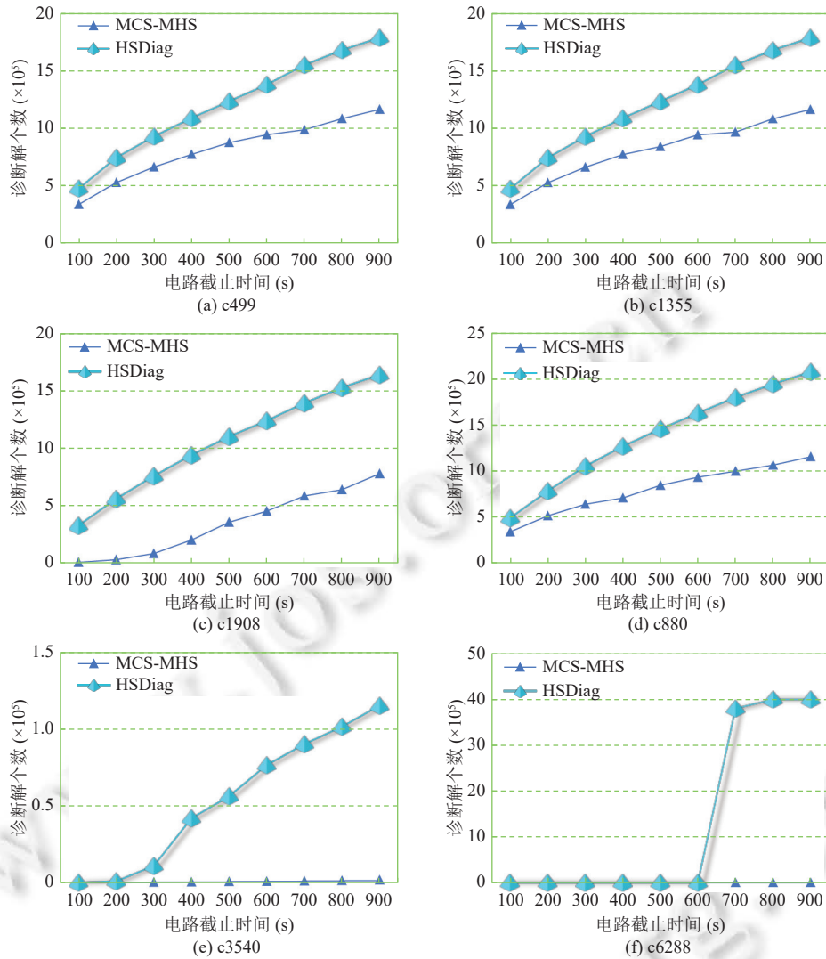
图 10 HSDiag 与 MCS-MHS 算法在 ISCAS-85 电路实验比较
