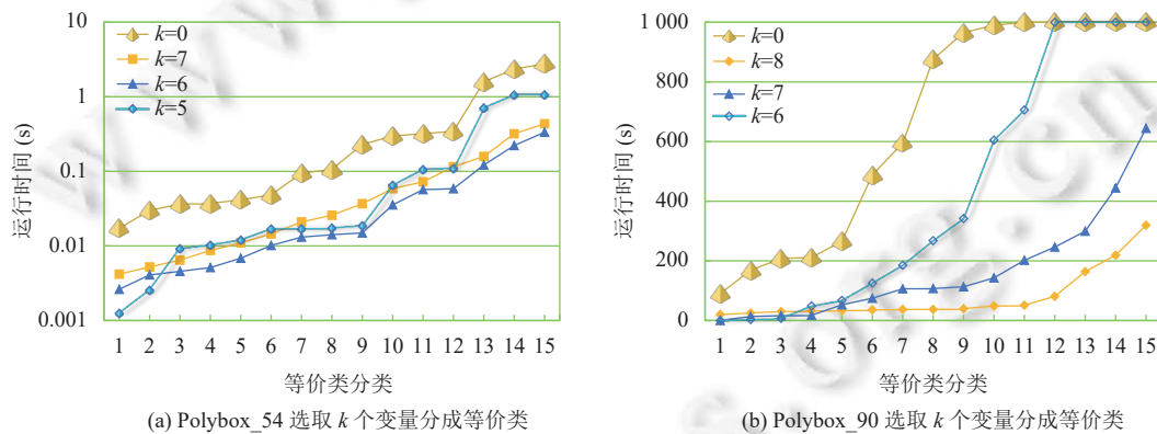
图 12 在 Polybox 电路中的等价类比较
