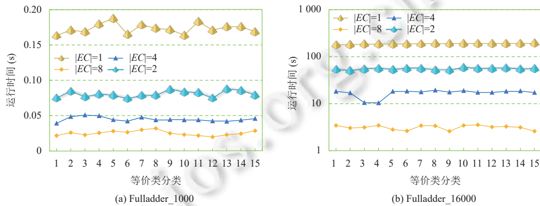
图 11 在 Fulladder 电路中的等价类比较
