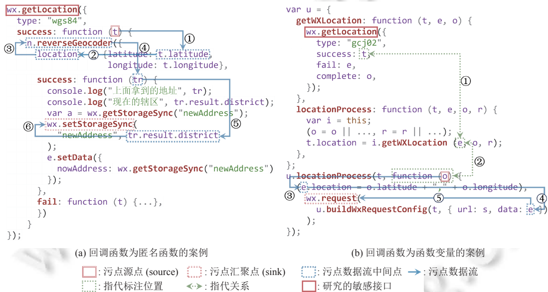
图 7 对回调函数形式返回数据接口的污点分析测试案例
