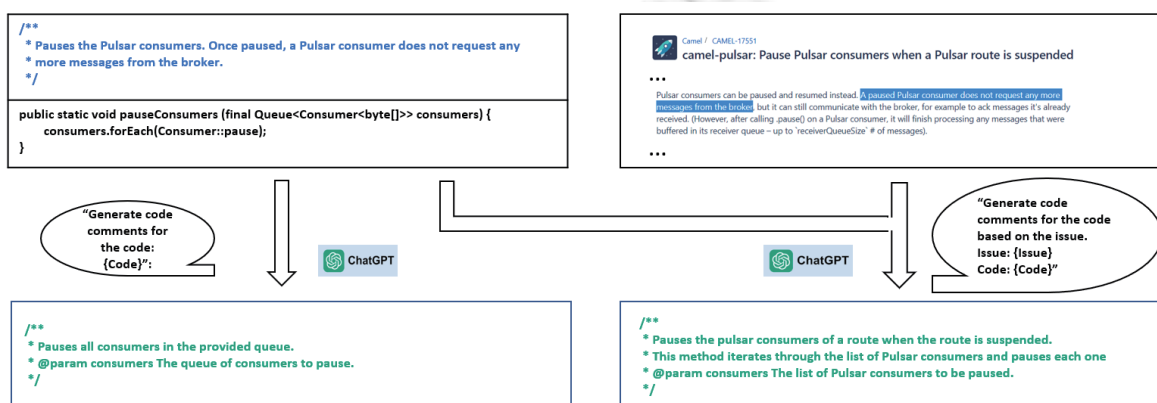
图2 Apache Camel 项目中一条补充性代码注释以及 ChatGPT 利用代码或 Issue 生成的注释
