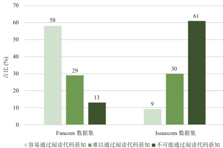
图4 Funcom 数据集与 Issuecom 数据集对比
