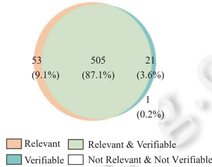
图 12 人工参考注释的代码相关性和 Issue 可验证性评价结果
