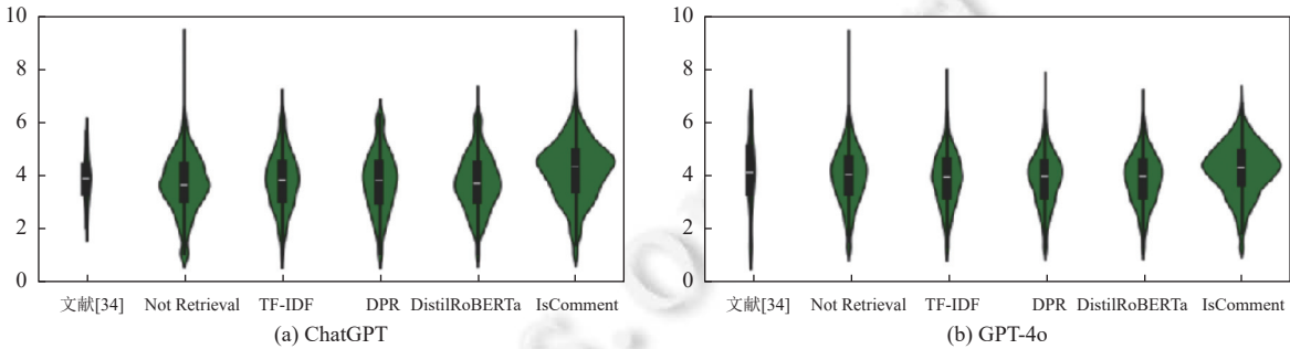
图 16 生成注释的补充性情况
