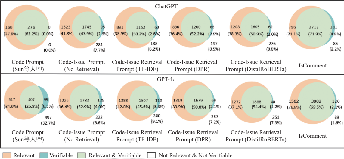
图 15 不同方法生成注释的代码相关性和 Issue 可验证性情况
