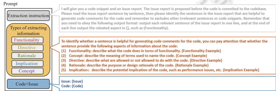
图 7 信息抽取阶段的 Prompt
