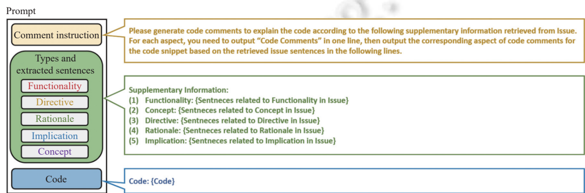
图 8 注释生成阶段的 Prompt
