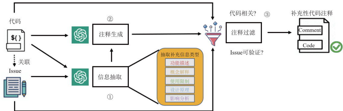
图 6 基于 Issue 检索增强语言模型的补充性代码注释生成方法框架
