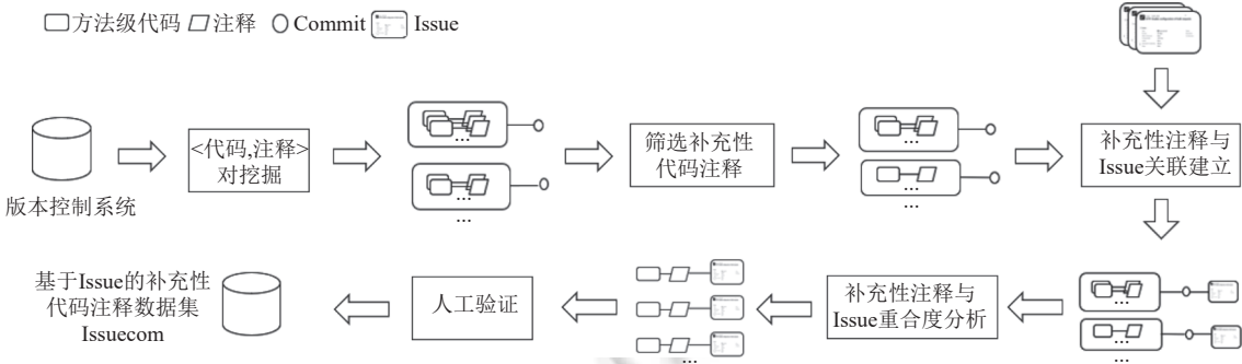
图 3 基于 Issue 的补充性代码注释收集流程
