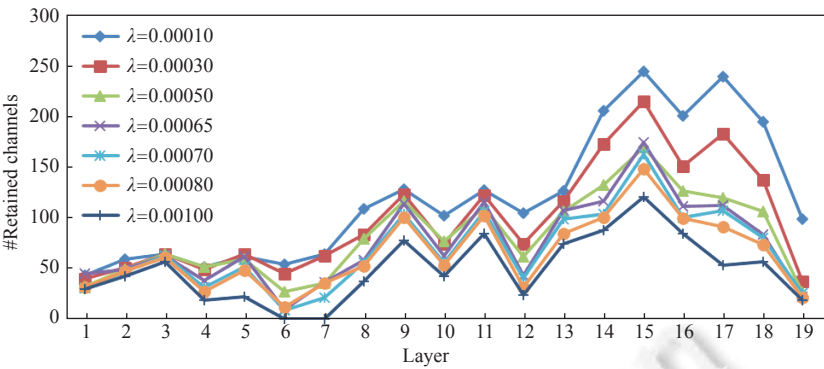
图3 CIFAR-10数据集上二值网络在不同正则化系数λ下的通道数结果
