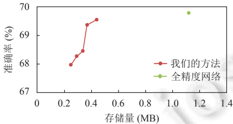
图 5 CIFAR-100 数据集上我们的方法得到的二值神经网络和全精度网络对比
