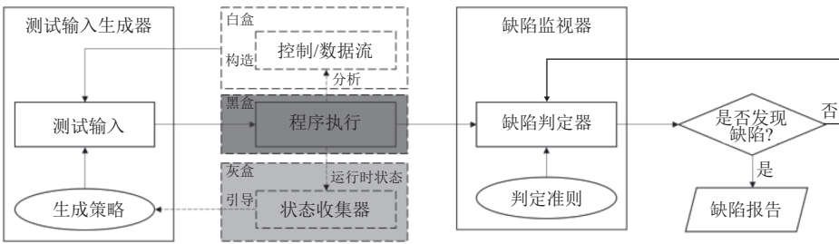
图 1 动态测试一般流程
