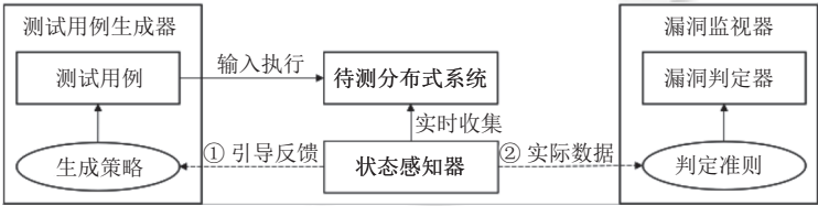
图 5 分布式系统动态测试核心流程
