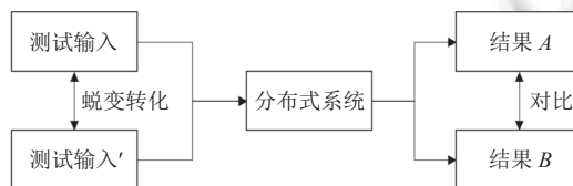
图 10 分布式系统蜕变测试示意图
