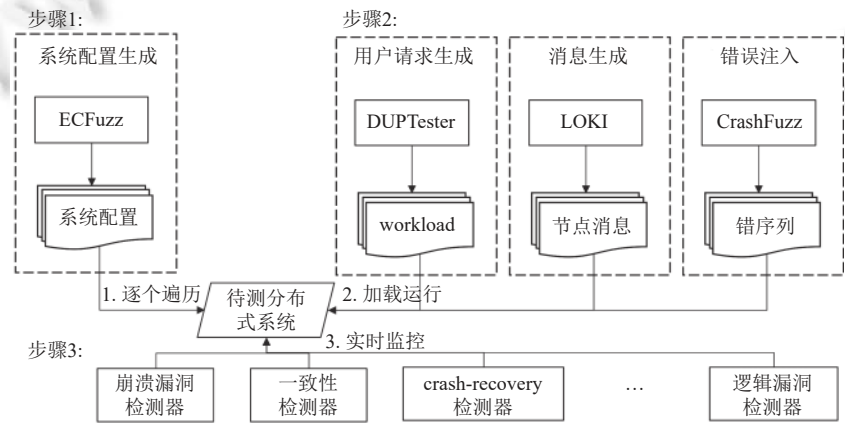
图 15 MultiGen 测试流程
