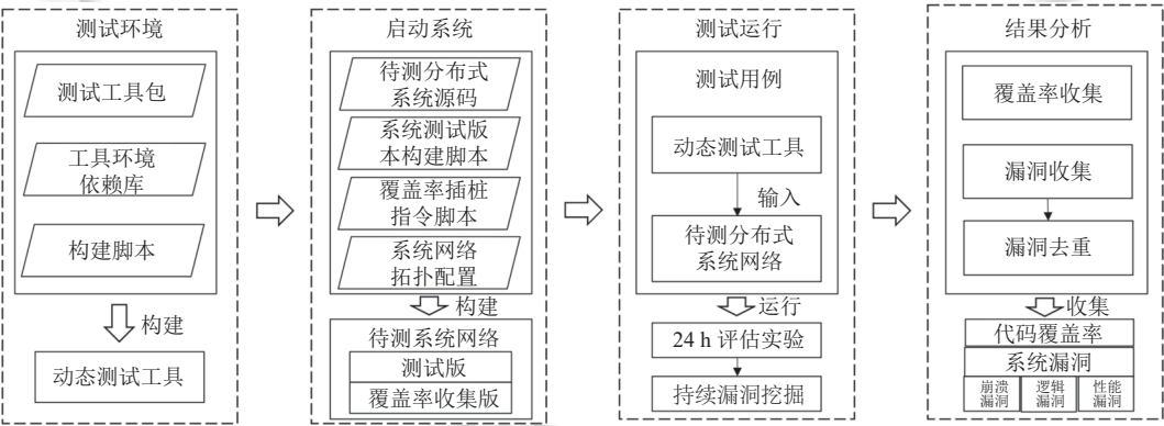
图 12 实验的测试过程
