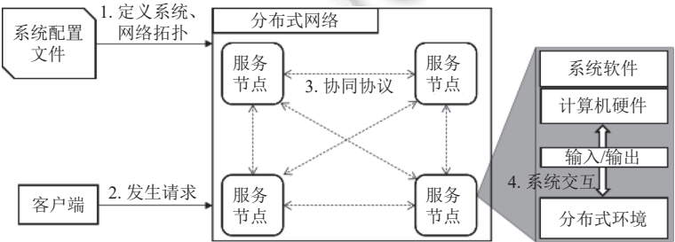
图 2 分布式系统一般运行流程
