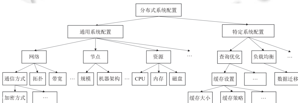
图 4 分布式系统一般配置模型
