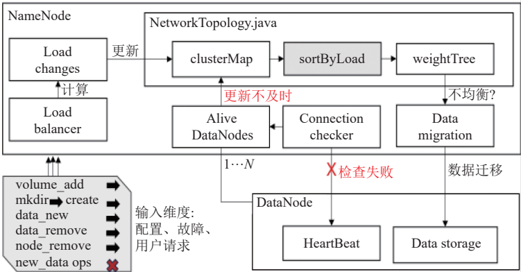
图 13 缺陷 HDFS-13279 的主要触发流程
