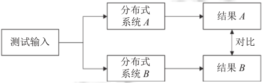
图 9 分布式系统差分测试示意图
