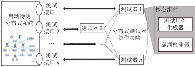
图 3 分布式系统动态测试一般架构
