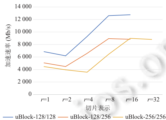
图 9 uBlock 算法不同切片表示下的加密性能
