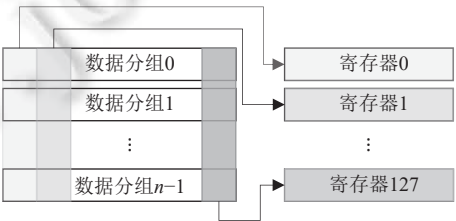
图 3 比特切片示例图
