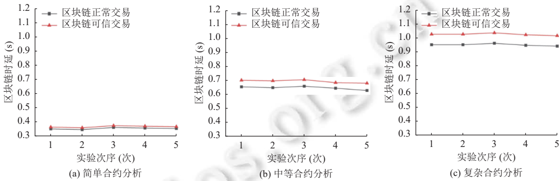
图 6 智能合约调用时延分析
