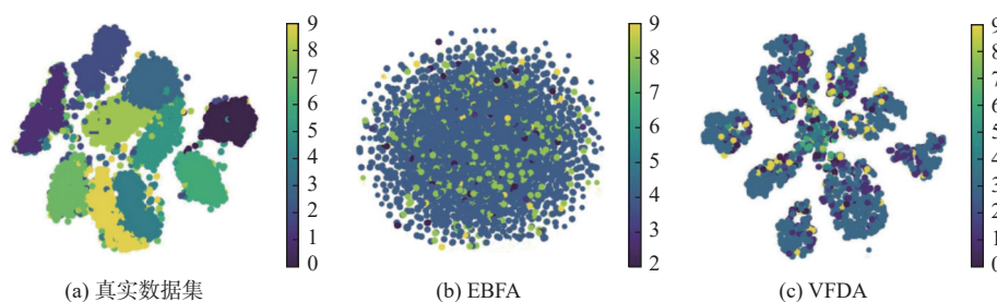
图4 在 CIFAR-10 数据集上, 原始数据、EBFA 生成的查询样本和 VFDA 生成的查询样本的 T-SNE 图
