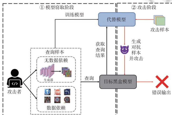
图1 模型窃取攻击中模型窃取阶段及攻击阶段示意图
