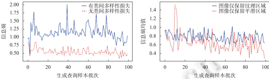
图 6 类间多样性损失和不同解码器对样本信息熵的影响
