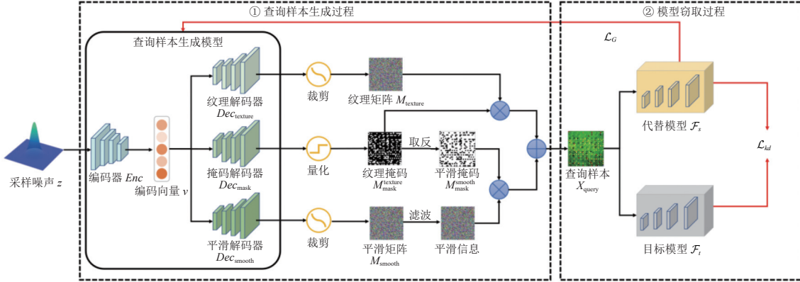
图 2 基于视觉特征解耦的模型窃取攻击方法总体框架图
