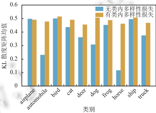
图 7 类内多样性损失对同一类别内样本 KL 散度的影响
