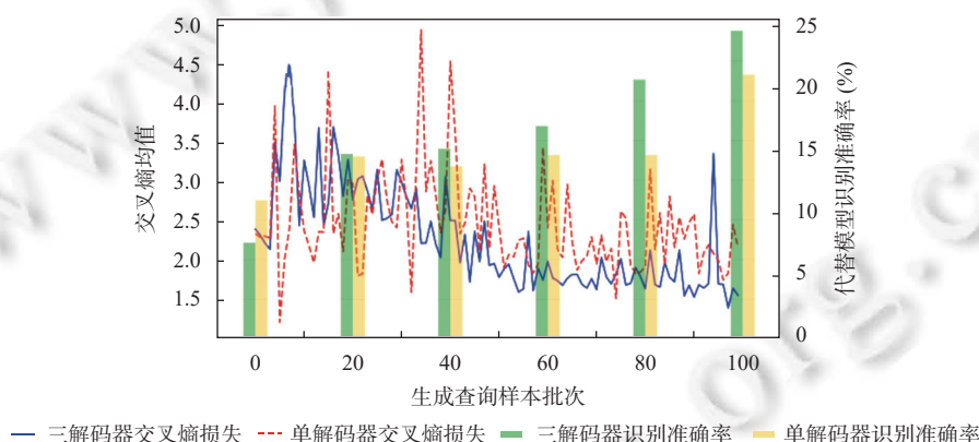
图5 不同生成器架构在模型窃取过程中对代替模型训练交叉熵和识别准确率的影响
