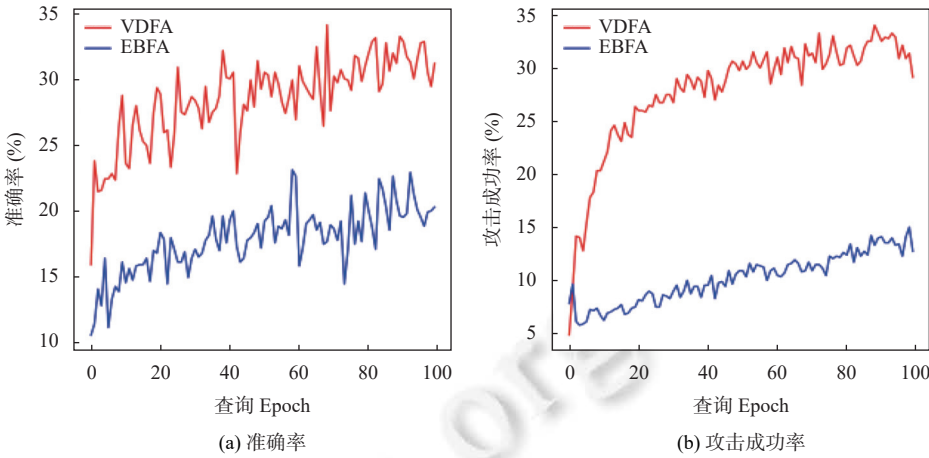
图 3 在 CIFAR-10 数据集上的模型窃取过程中模型收敛速度对比
