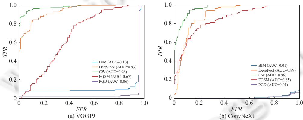
图 9 ImageNet 上不同攻击下单阈值检测器的检测性能
