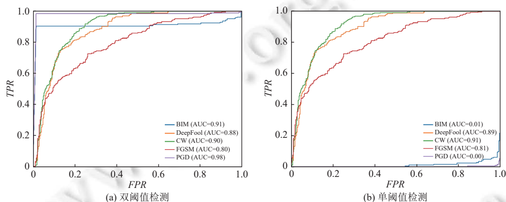
图8 CIFAR-10 上不同攻击下检测器的检测性能
