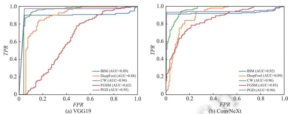
图7 ImageNet 上不同攻击下检测器的检测性能
