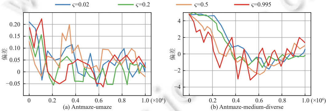
图 5 不同动作权重系数的 DMEM 学习曲线图
