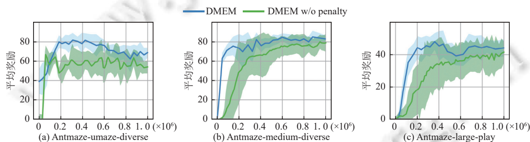
图 7 DMEM 和没有动作惩戒项的 DMEM 的算法对比学习曲线图
