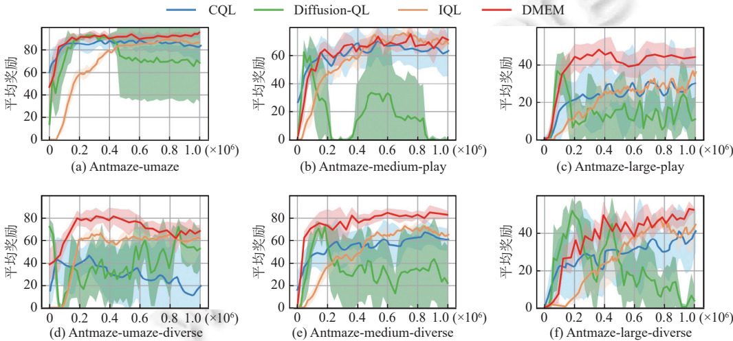
图 4 DMEM 和其他离线强化学习算法学习曲线图
