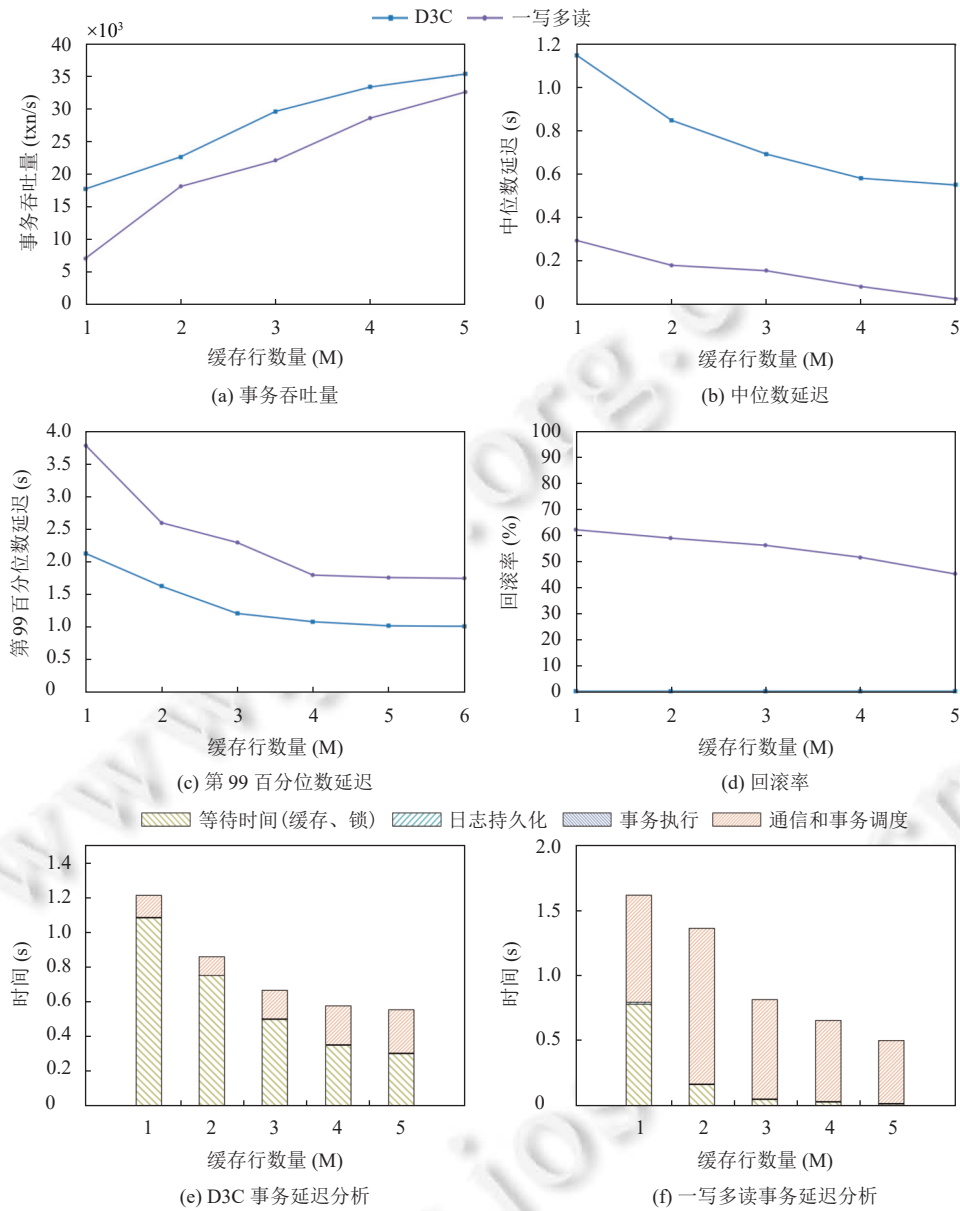
图 12 TPC-C 缓存行数量测试
