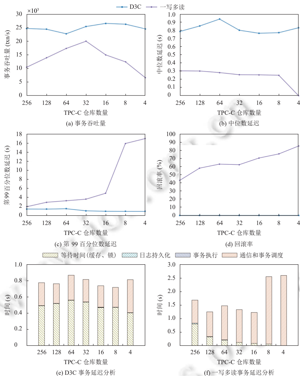
图 13 TPC-C 仓库数量测试
