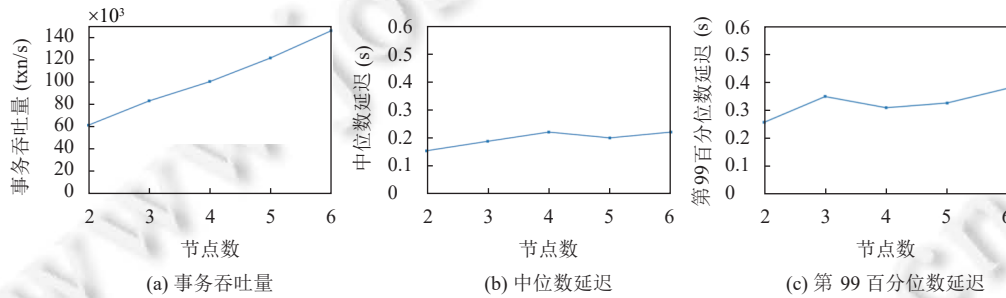
图 16 D3C 的可扩展性测试
