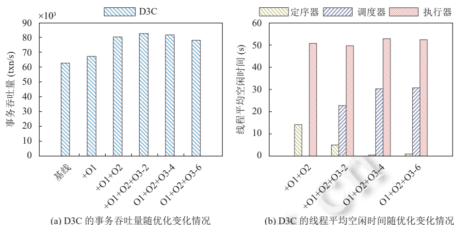
图 11 D3C 优化效果测试
