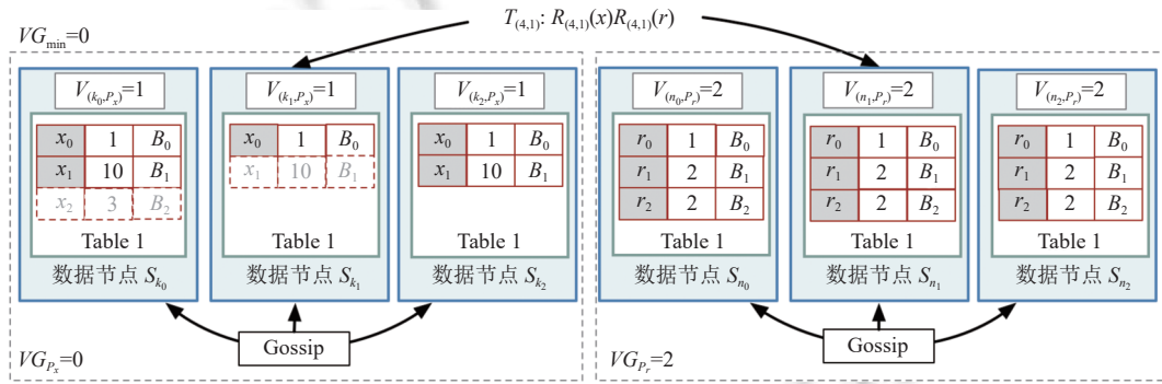
图 6 基于数据一致性点的只读事务优化
