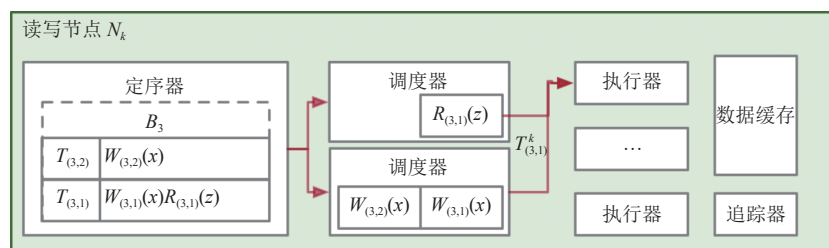
图7 多线程加锁
