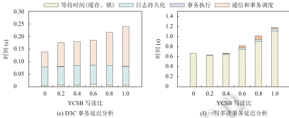
图 15 YCSB 写读比测试 (续)
