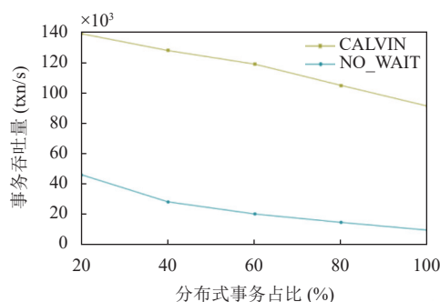
图1 分布式数据库场景下确定性并发控制和基于 2PC 的并发控制性能对比
