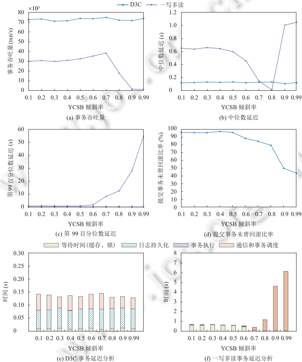
图 14 YCSB 倾斜率测试
