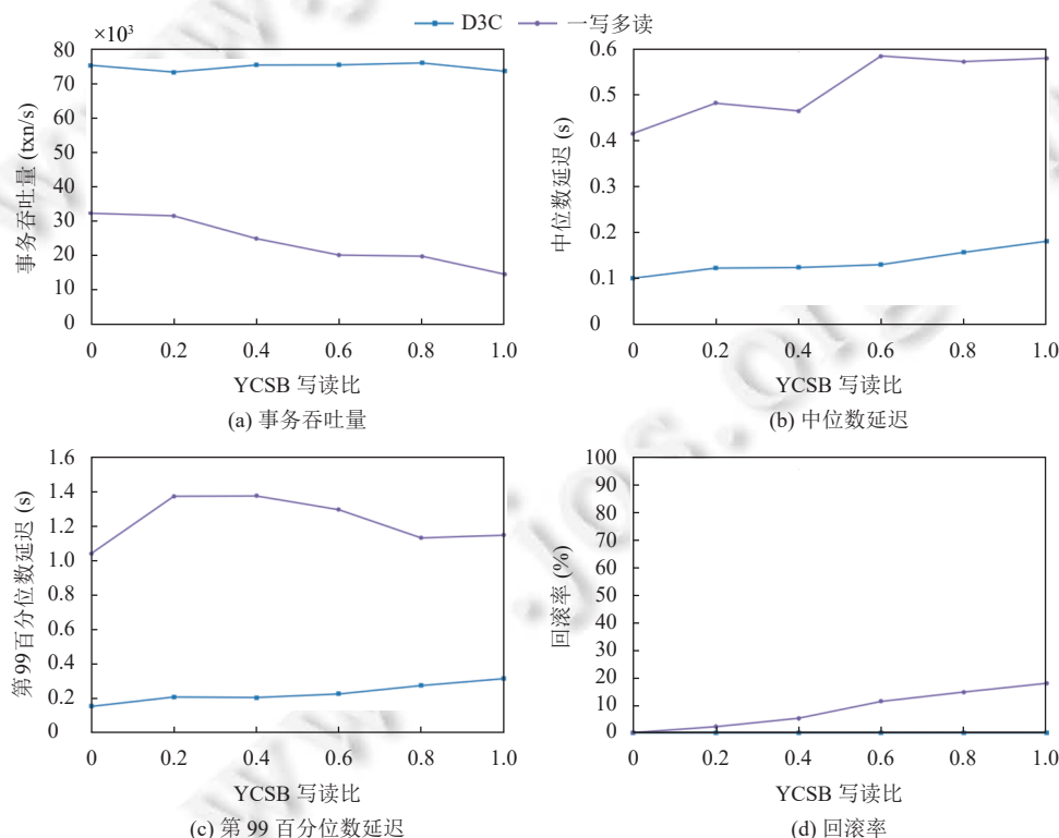
图 15 YCSB 写读比测试
