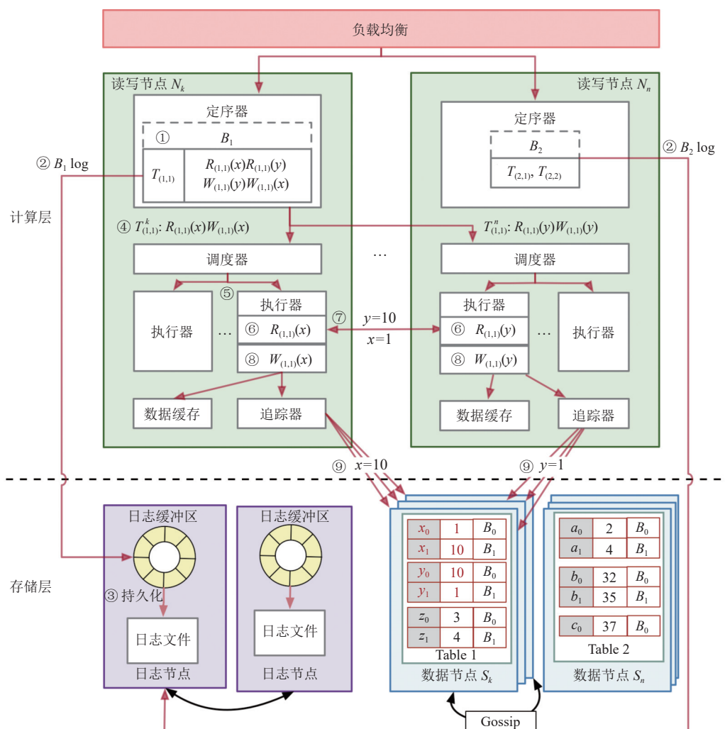
图4 云原生多写事务处理架构 D3C
