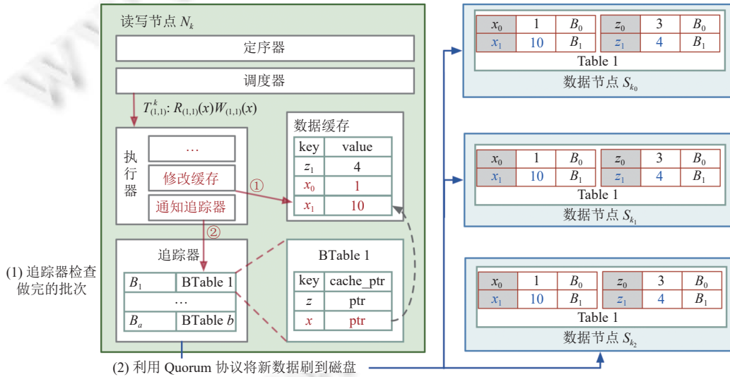
图 5 D3C 持久化机制
