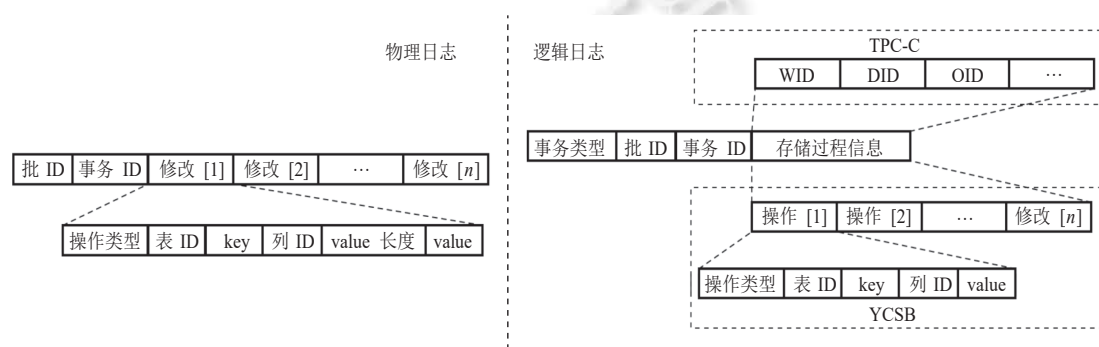
图 10 日志结构
