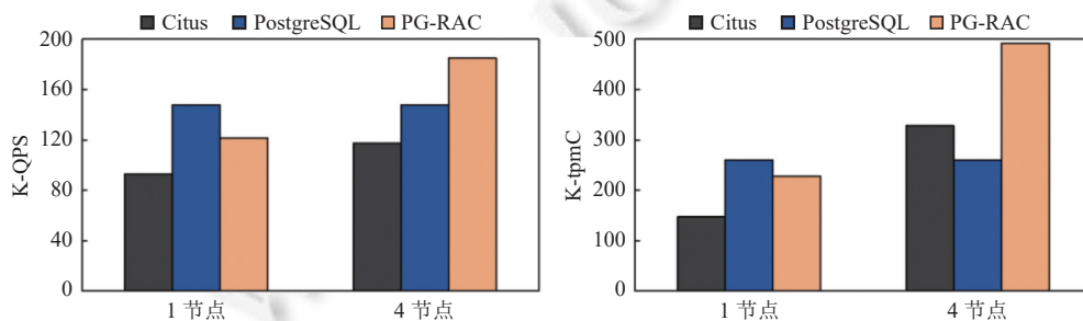
图 9 PG-RAC 与其他数据库对比测试
