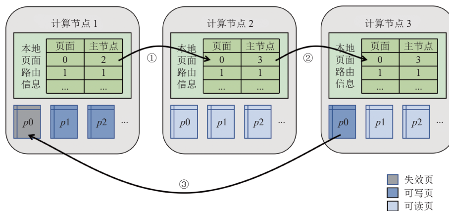
图 3 链式路由机制
