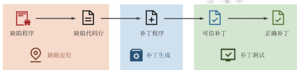
图 7 软件缺陷自动修复技术机制
