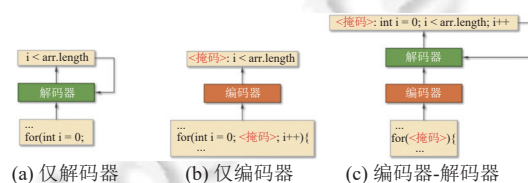
图3 大语言模型的3种架构
