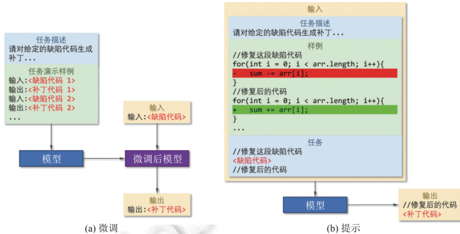
图4 模型应用于下游任务的方式
