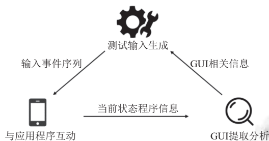
图6 GUI 自动化测试总体流程
