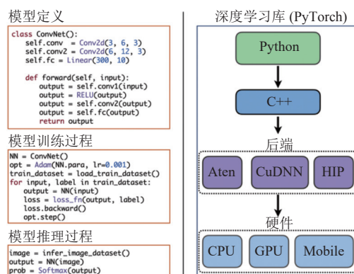
图 5 深度学习模型与深度学习库概览
