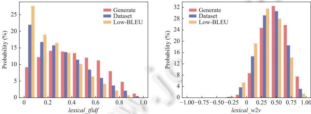
图 8 3 个注释集合在 lexical_tfidf 、 lexical_w2v 上的分布
