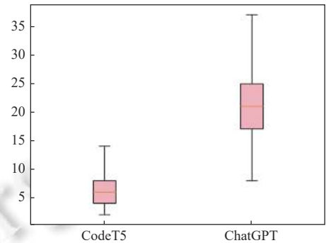
图 13 CodeT5 与 ChatGPT 生成注释的长度分布
