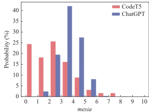
图 12 CodeT5 与 ChatGPT 生成注释在 mesia 指标上的分布
