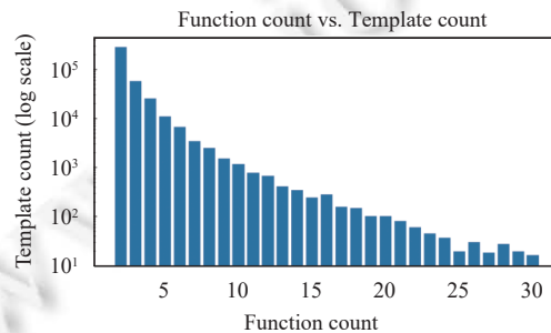
图 3 模板的函数融合度
