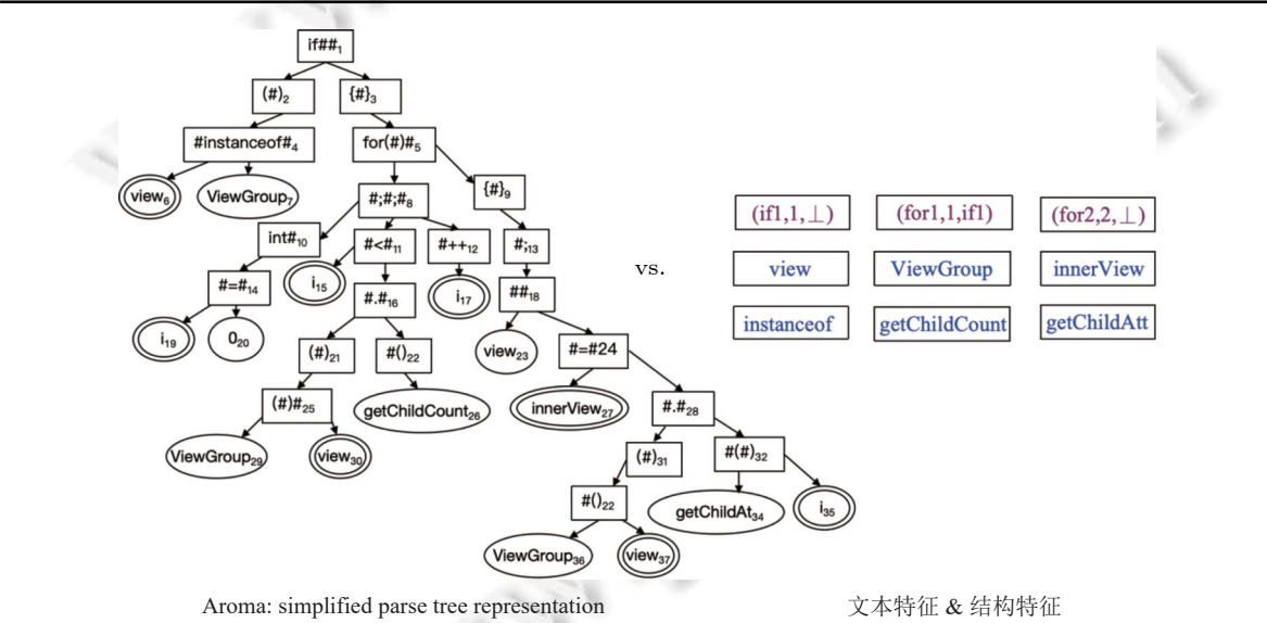
图 2 特征表示方法对比
