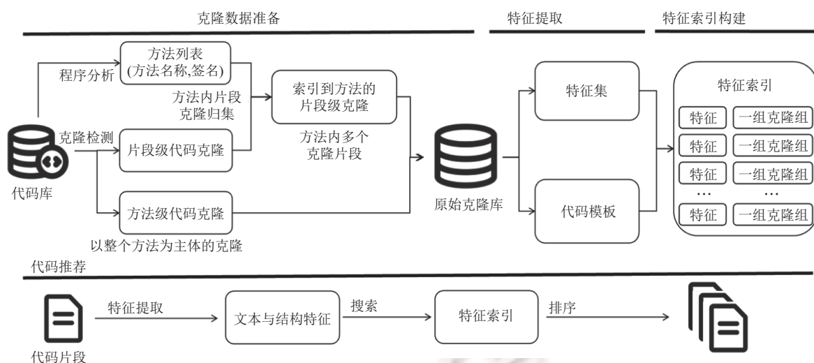
图1 CodeSculptor 架构图
