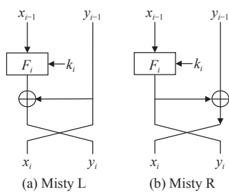
图 2 Misty L 和 Misty R 结构
