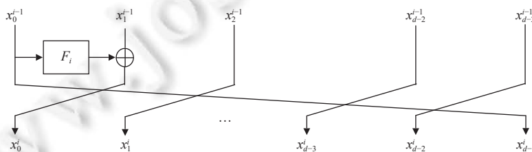
图 4 第 i 轮 Type-1 型广义 Feistel 结构
