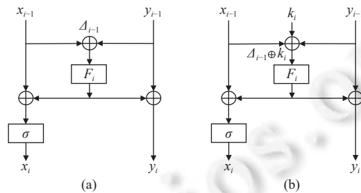
图 1 Lai-Massey 结构
