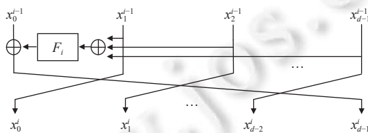
图 5 第 i 轮类 SMS4 广义 Feistel 结构
