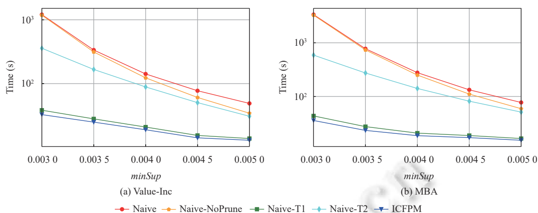
图3 算法在 \min Sup 变化时运行时间比较
