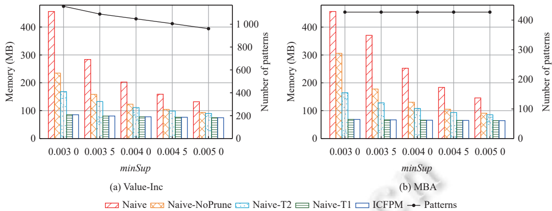
图7 算法在 minSup 变化时空间开销比较
