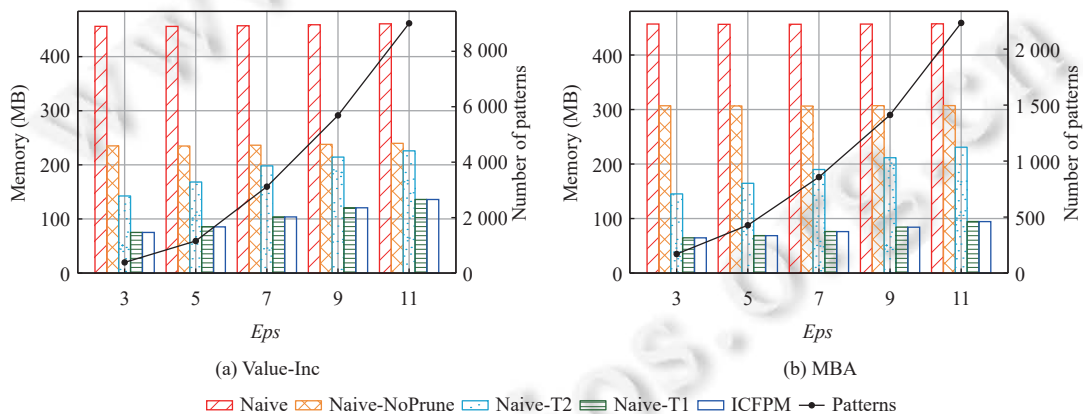
图8 算法在 Eps 变化时空间开销比较
