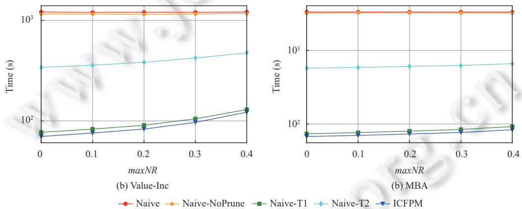
图 6 算法在 maxNR 变化时运行时间比较
