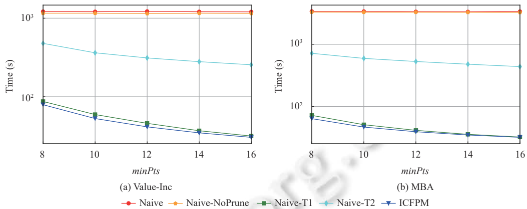
图 5 算法在 minPts 变化时运行时间比较
