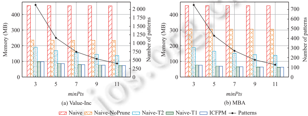
图 9 算法在 minPts 变化时空间开销比较
