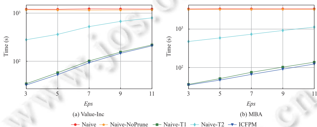
图4 算法在 Eps 变化时运行时间比较
