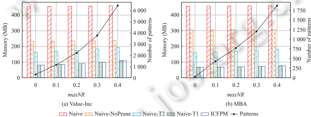
图 10 算法在 maxNR 变化时空间开销比较
