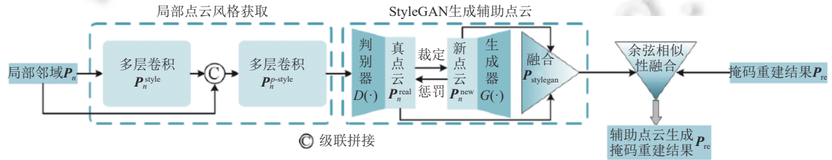
图 4 基于 StyleGAN 的辅助点云生成模型
