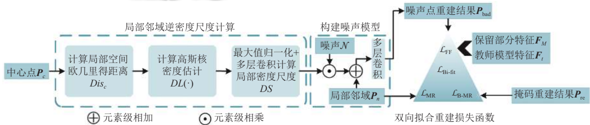
图3 逆密度尺度指导下的“坏教师”模型
