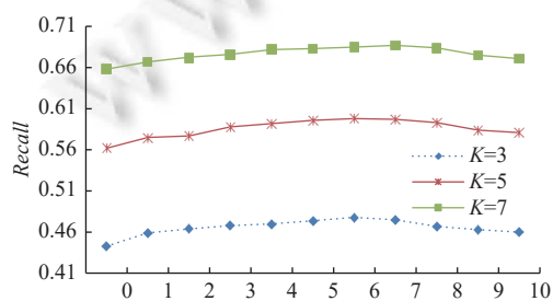
图 9 不同 K 值下的 Recall 对比
