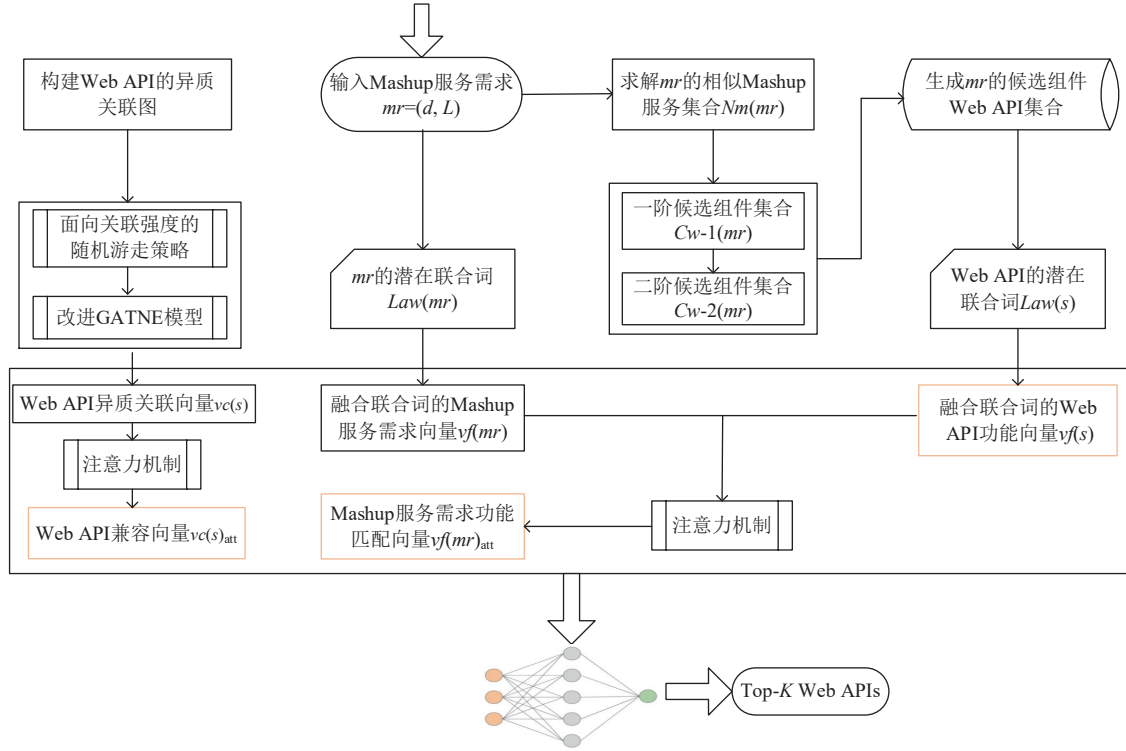
图5 研究框架
