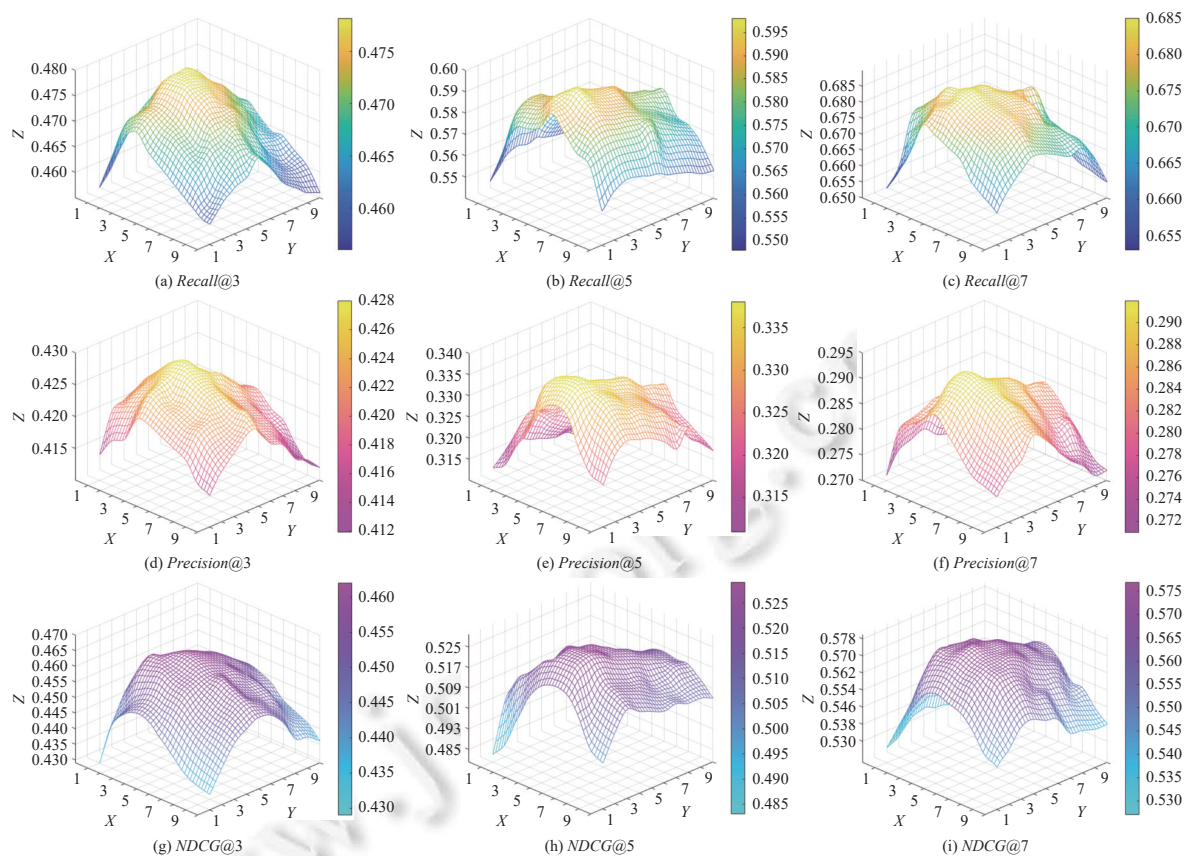
图 8 采样邻居数量指标图
