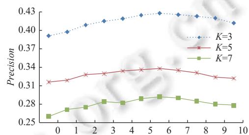
图 10 不同 K 值下的 Precision 对比
