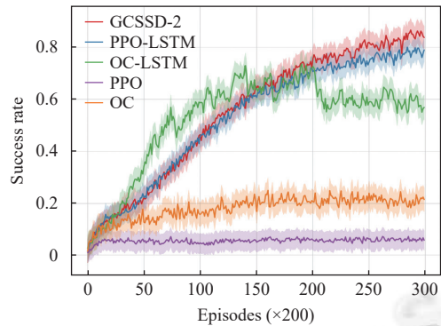
图 6 网络世界训练曲线
