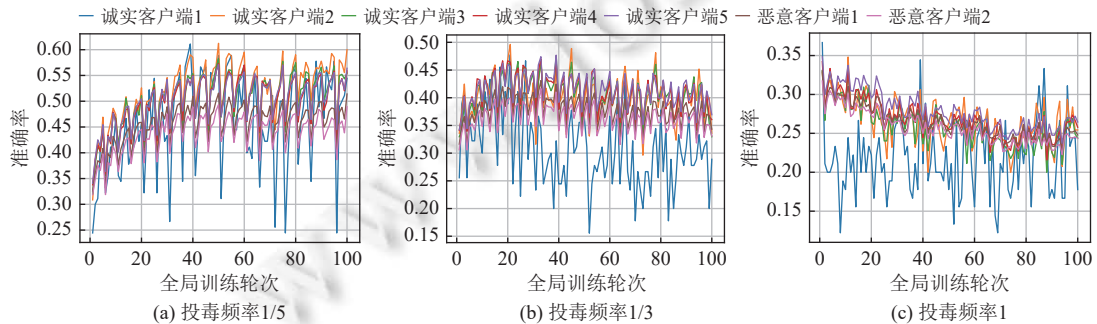
图 5 恶意终端节点数量为 6 时, 不同投毒频率在 CIFAR10 上的实验结果
