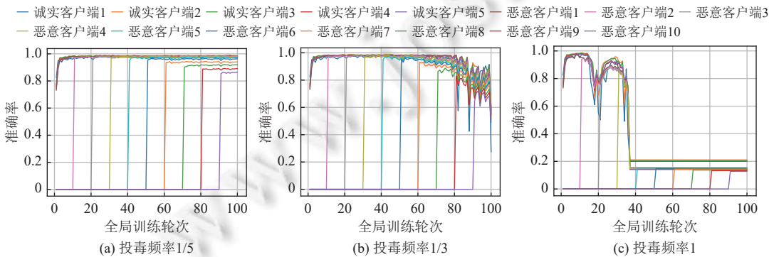
图 9 在 MNIST 上, 不开启特征图甄别防御的模型准确率对比图
