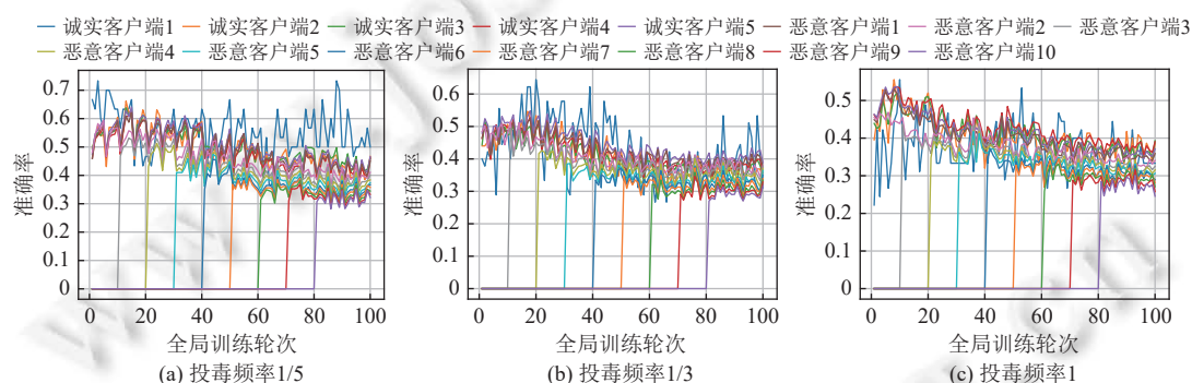
图 11 在 CIFAR10 上, 不开启特征图甄别防御的模型准确率对比图
