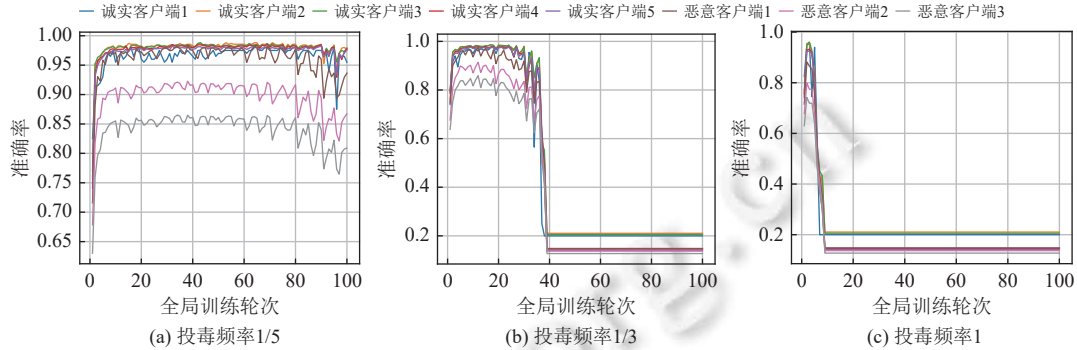
图 3 恶意终端节点数量为 10 时, 不同投毒频率在 MNIST 上的实验结果
