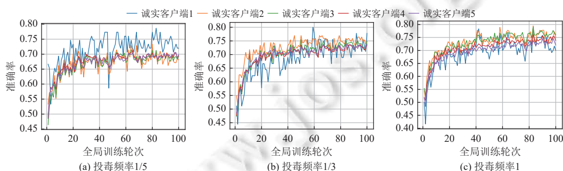
图 12 在 CIFAR10 上, 开启特征图甄别防御的模型准确率对比图
