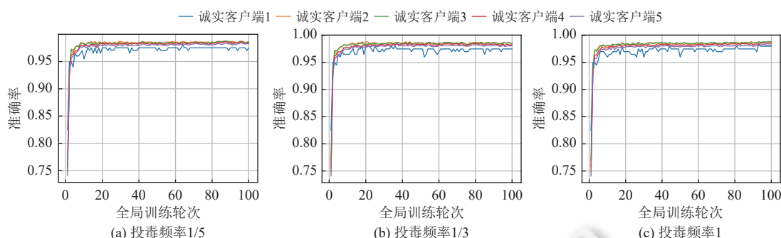
图 10 在 MNIST 上, 开启特征图甄别防御的模型准确率对比图
