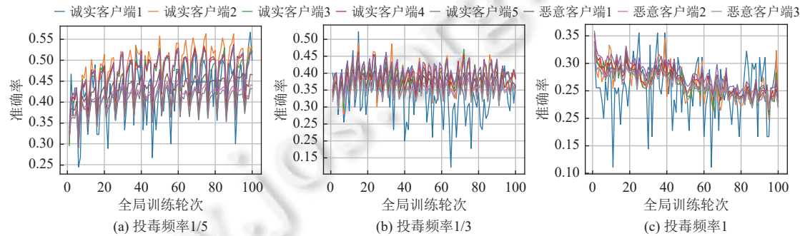
图 6 恶意终端节点数量为 10 时, 不同投毒频率在 CIFAR10 上的实验结果
