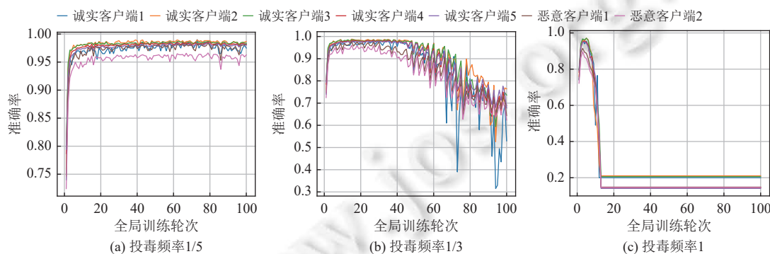
图 2 恶意终端节点数量为 6 时, 不同投毒频率在 MNIST 上的实验结果
