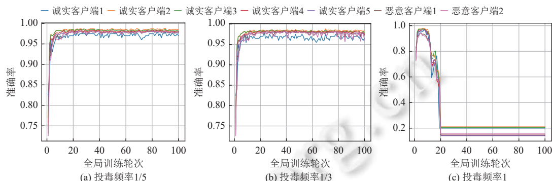
图 1 恶意终端节点数量为 2 时, 不同投毒频率在 MNIST 上的实验结果
