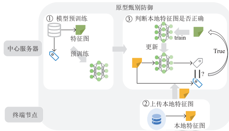
图 8 原型甄别防御流程
