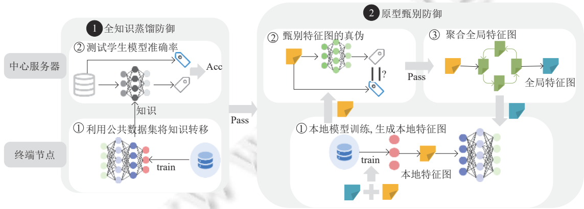
图 7 De-FMPA 防御流程
