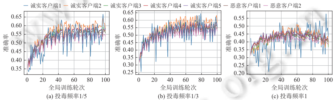
图 4 恶意终端节点数量为 2 时, 不同投毒频率在 CIFAR10 上的实验结果
