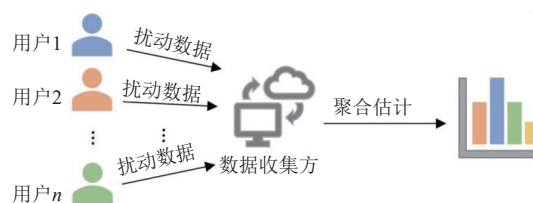
图 1 本地差分隐私模型框架
