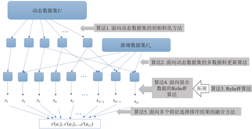
图1 算法框架图
