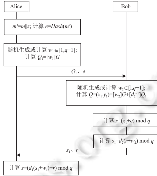
图1 基于乘法密钥拆分的两随机数两方门限计算方案框架
