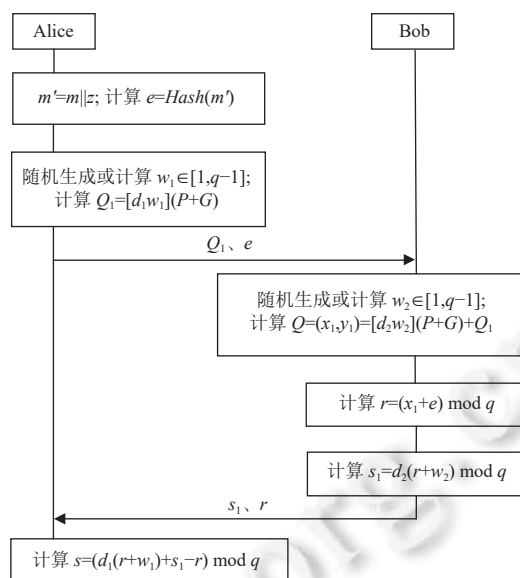
图3 基于加法密钥拆分的两随机数两方门限计算方案框架
