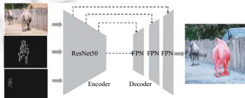
图7 骨架映射网络结构图
