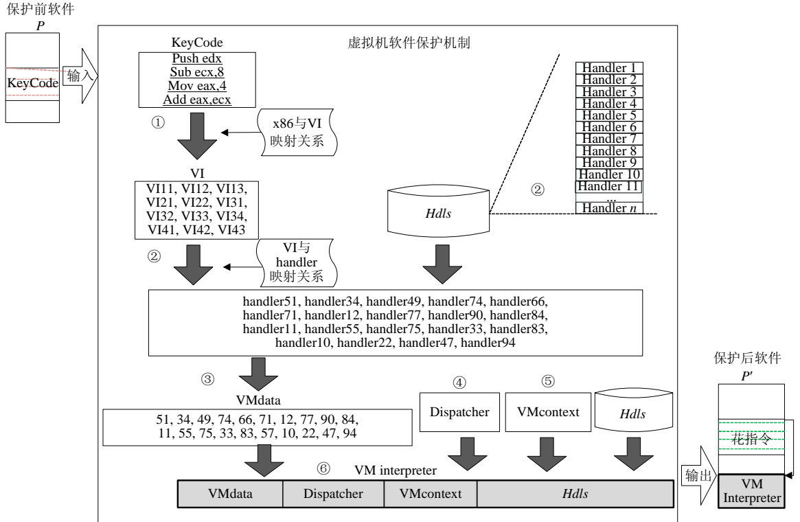
Fig.2 Mechanism of virtual machine protection 图 2 虚拟机软件保护机制
