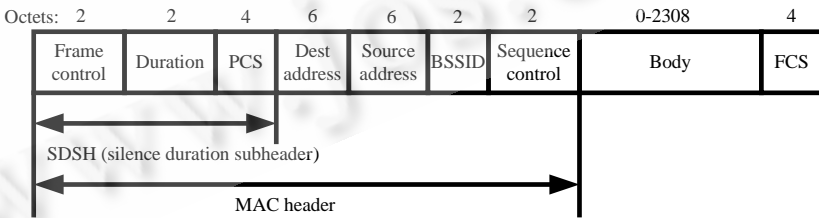
Fig.9 MAC data frame for DATA in PCSMAC 图 9 PCSMAC 中数据包 DATA 的 MAC 帧结构
