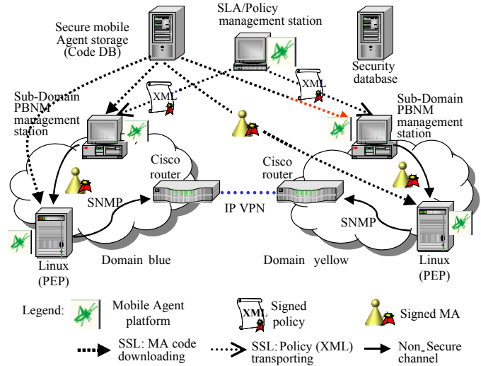
Fig.3 Safe inter-domain virtual private network management system 图 3 安全的域间虚拟专用网络管理系统
