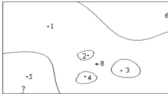
Fig.2 Surface TTP distribute graph
