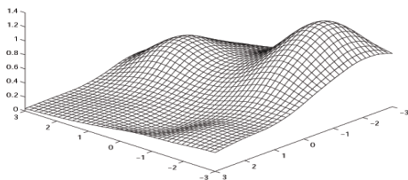
Fig.3 Surface G(u, v) 图 3 曲面 G(u, v)
