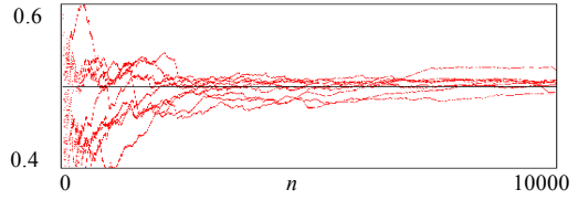
Fig.4 \alpha(M, x_0, n) of different key x_0 , when M=0^n 图4 不同密钥 x_0 的分布函数 \alpha(M, x_0, n) , M=0^n
