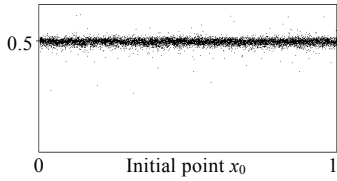
Fig.3 \alpha(M, x_0, n) , when n=10000 and M=0^n 图3 分布函数 \alpha(M, x_0, n) , n=10000 , M=0^n
