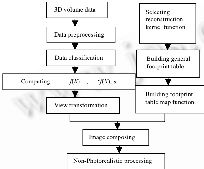
三维体数据, 数据预处理, 数据分类, 计算, 视觉变换, 选择重构核, 建立通用足迹表, 建立足迹映射函数, 图像组合, 非真实感绘制.
