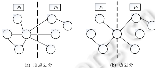
图 2 顶点划分与边划分
