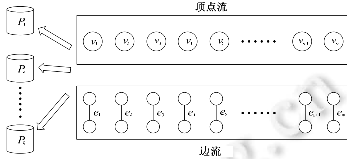
图 6 流式图划分算法思路框架图
