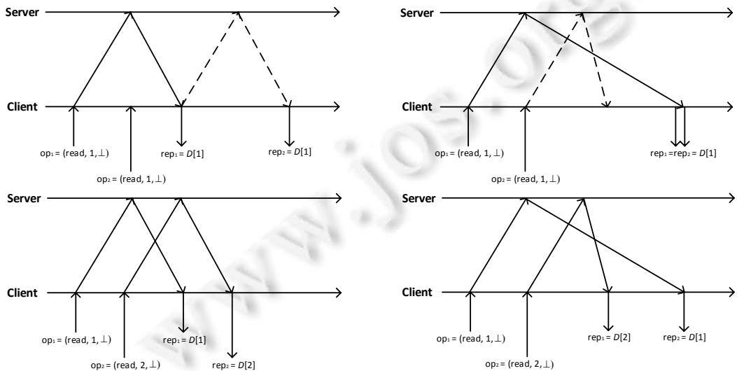
(a) 在 ObliviStore 中对相同数据块访问的响应时间(上图) 对 不同数据块访问的响应时间(下图) (b) 在 CURIOUS 中对相同数据块访问的响应时间(上图) 对 不同数据块访问的响应时间(下图)
