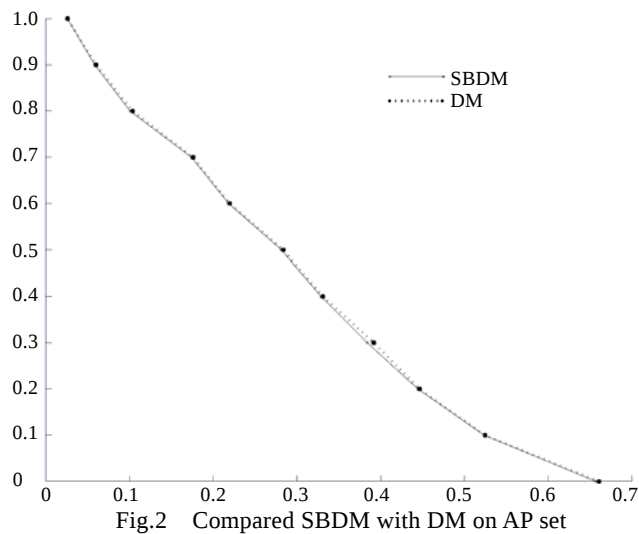
图 2 AP 数据集 SBDM 与 DM 的比较
