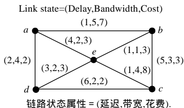
Fig.1 Weighted graph network model 图 1 有权图网络模型
